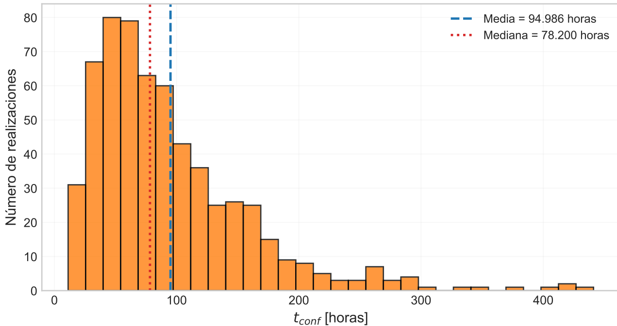
Distribución de t_{conf} (T = 4 K, N = 600)
