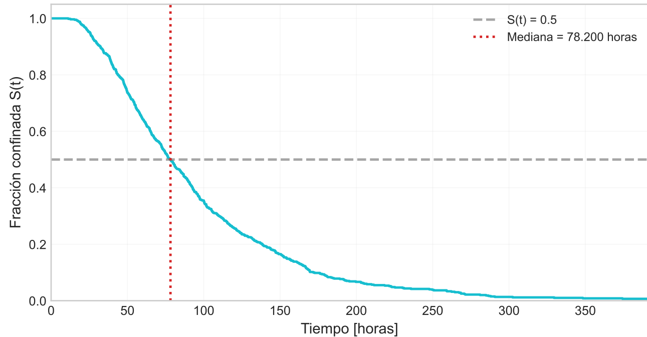
Curva de supervivencia S(t) ( T = 4 K)
