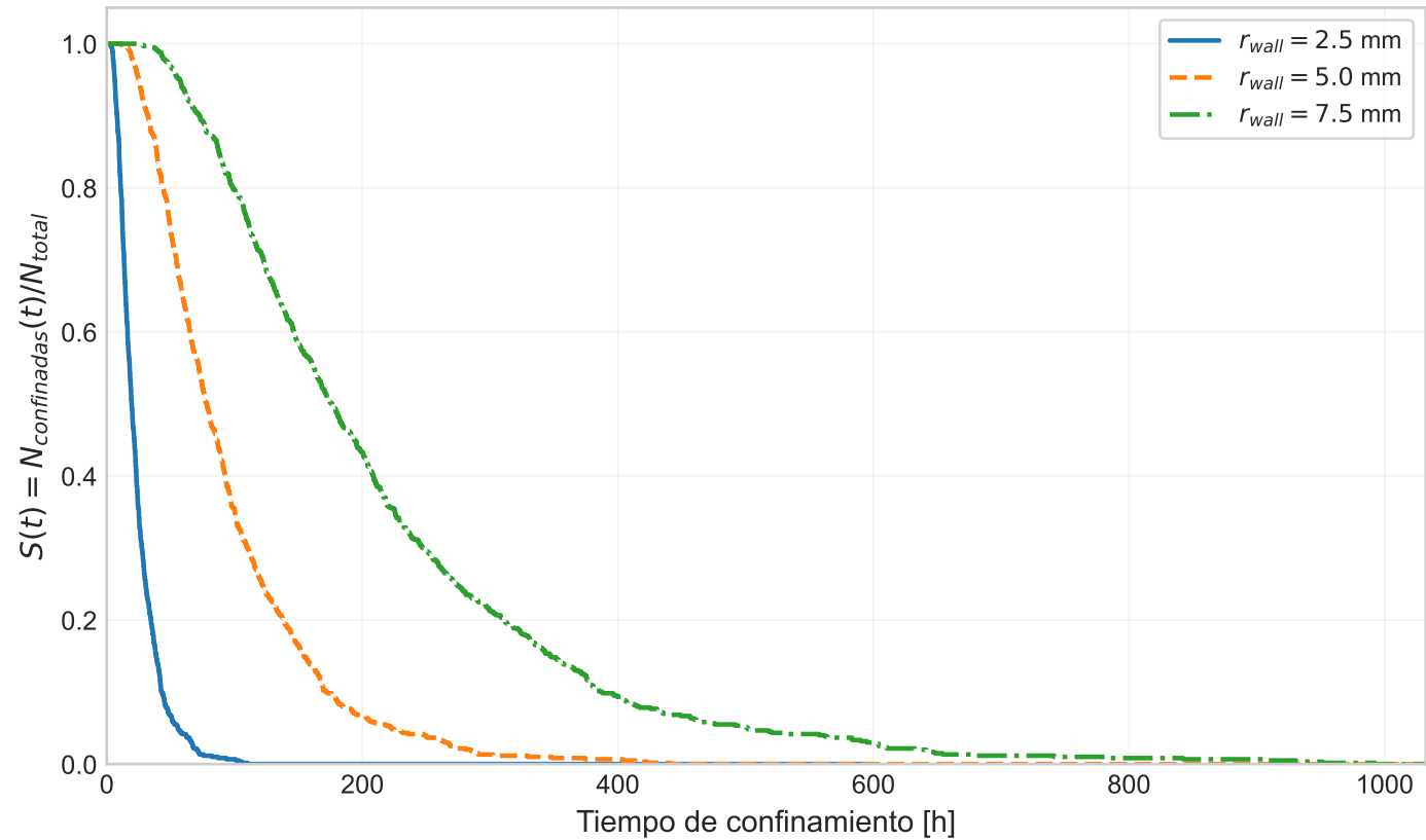
Sensibilidad del tiempo de confinamiento al radio efectivo, T = 4 K
