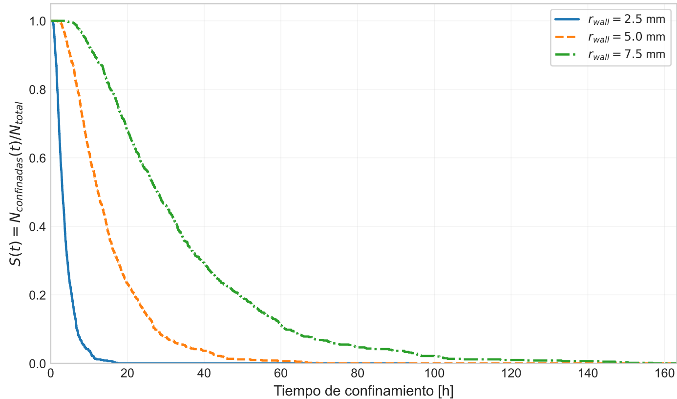
Sensibilidad del tiempo de confinamiento al radio efectivo, T = 0,1 K
