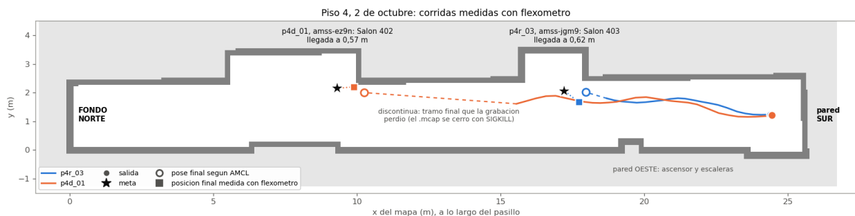
Figura 4.2. Dos misiones sobre hardware en el pasillo del piso 4, una por cada vehículo. La estrella es el destino del catálogo; el cuadrado, la posición final medida con flexómetro. El tramo a trazos de la corrida naranja es la parte final que la grabación perdió, no un salto del vehículo.
