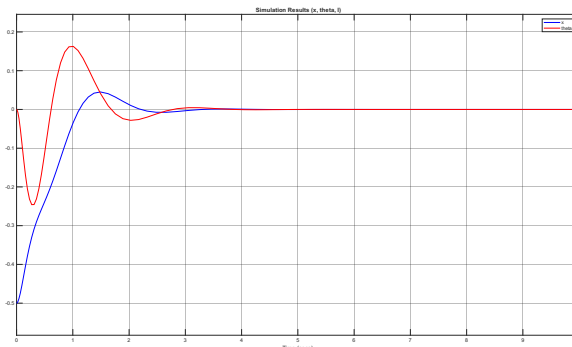
شکل ۳.۲ پاسخ زمانی موقعیت کالسکه و زاویه آونگ برای جابجایی ۵/۰ متر
