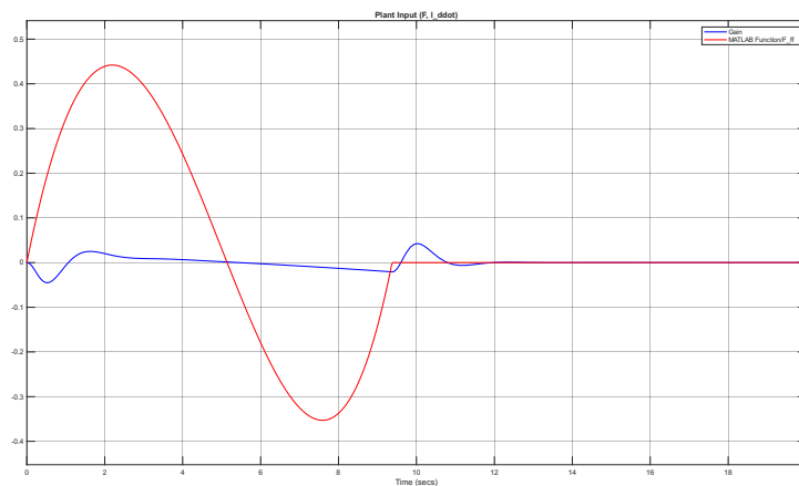
شکل ۱۲.۳ تفکیک سیگنال‌های کنترلی (فیدفورارد و فیدبک) در جابجایی ۵ متر
