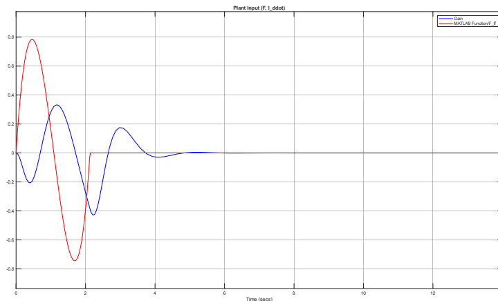
شکل ۹.۳ تفکیک سیگنال‌های کنترلی (فیدفورارد و فیدبک) در جابجایی ۰/۵ متر
