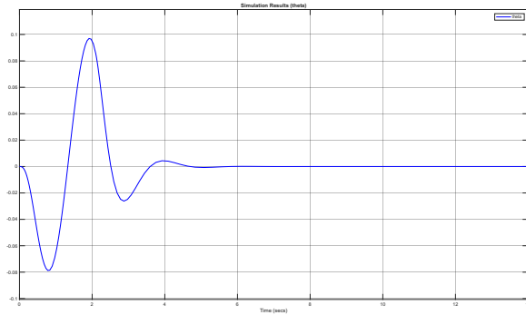
شکل ۸.۳ زاویه نوسان آونگ در جابجایی ۰/۵ متر
