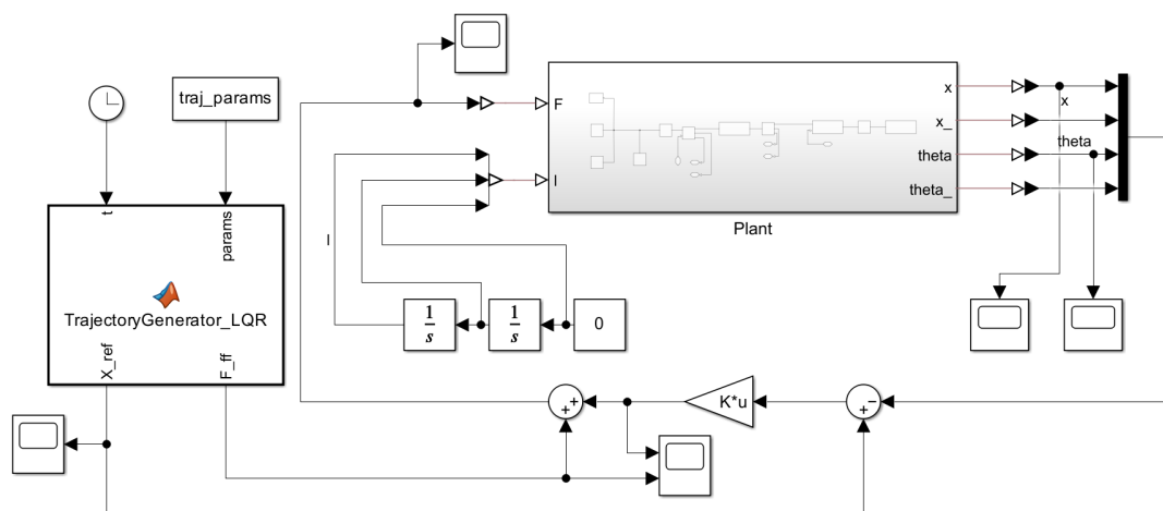
شکل ۶.۳ معماری یکپارچه کنترل کننده LQR مبتنی بر برنامه ریز مسیر و فیدفوروارد
