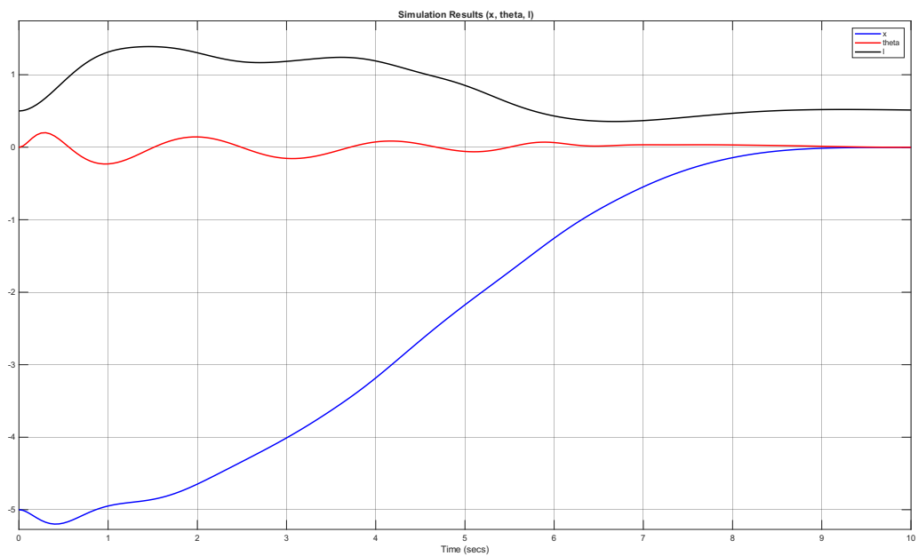
شکل ۱۱.۲ پاسخ زمانی موقعیت کالسکه، زاویه نوسان و طول کابل برای جابجایی ۵ متر
