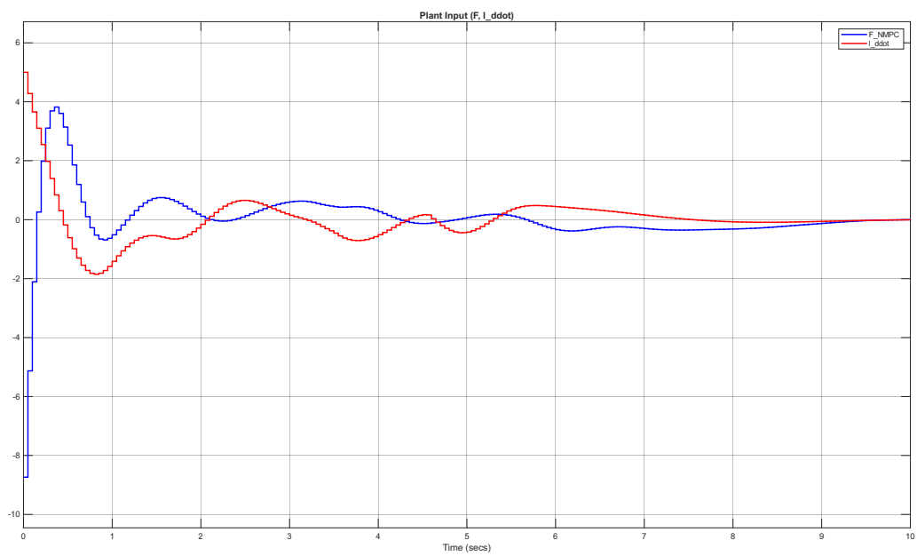
شکل ۱۲.۲ سیگنال‌های کنترلی اعمال شده به سیستم برای جابجایی ۵ متر
