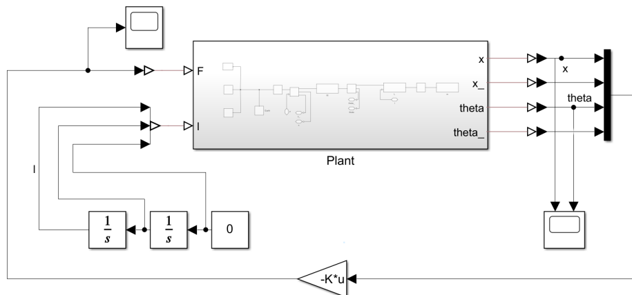
شکل ۲.۲ معماری حلقه بسته کنترل کننده خطی LQR با فرض طول کابل ثابت.
