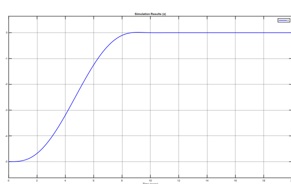
شکل ۱۰.۲ ردیابی موقعیت کالسکه در جابجایی 5 متر
