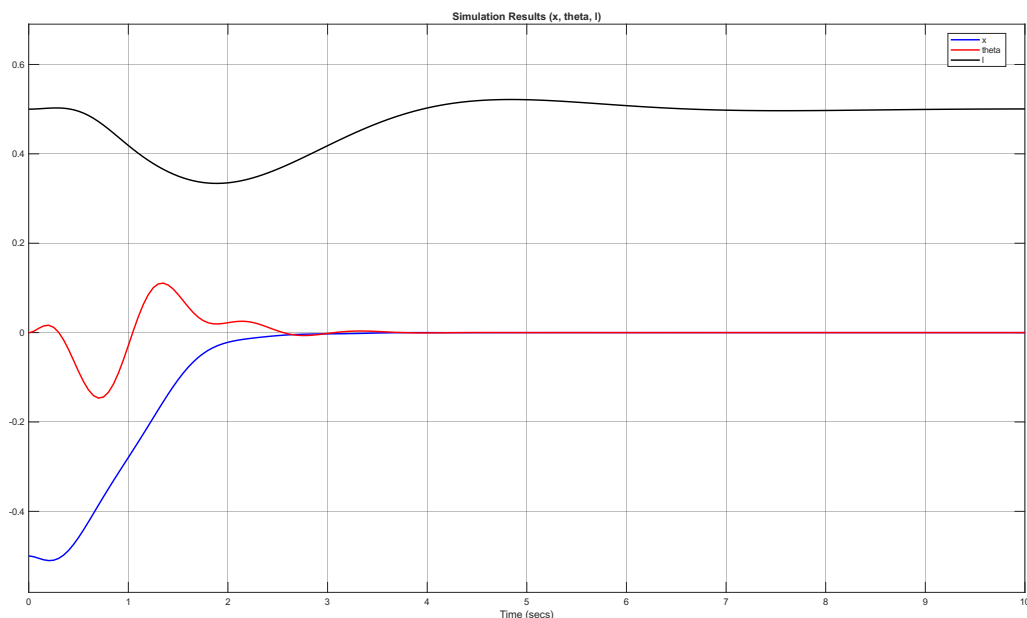
شکل ۱۴.۲ پاسخ زمانی موقعیت کالسکه، زاویه نوسان و طول کابل برای جابجایی 0.5 متر
