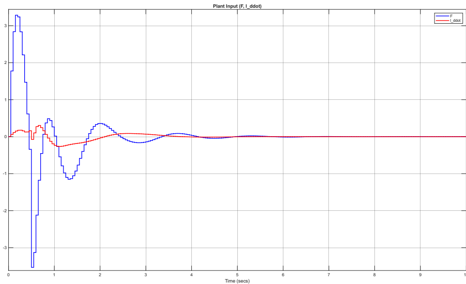
شکل ۱۱.۲ سیگنال‌های کنترلی اعمال شده به پلنت: نیروی کالسکه ( F ) و شتاب تغییر طول کابل ( \ddot{l} )
