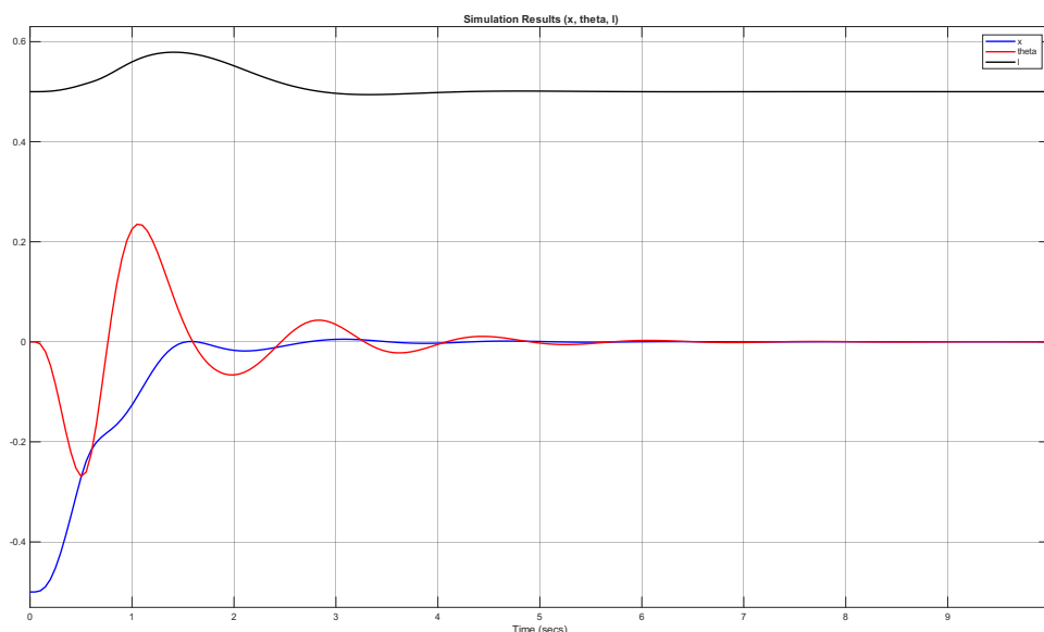
شکل ۱۰.۲ پاسخ زمانی موقعیت کالسکه، زاویه نوسان و طول کابل
