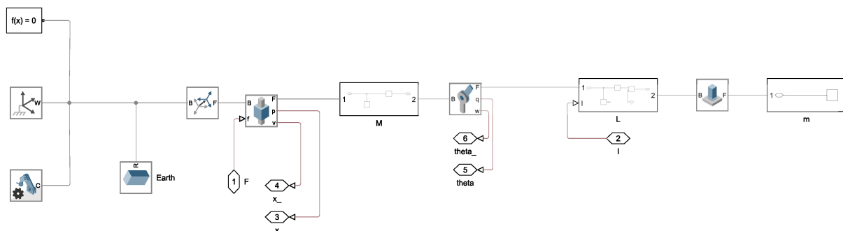
شکل ۸.۲ معماری داخلی مدل Simscape Multibody شامل مفاصل، بلوک‌های فیزیکی و زنجیره سینماتیکی
