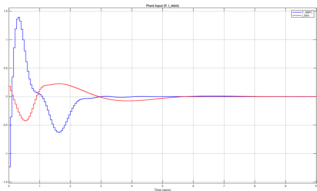
شکل ۱۵.۲ سیگنال‌های کنترلی اعمال‌شده به سیستم برای جابجایی 0.5 متر
