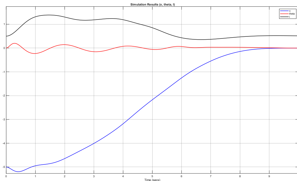
شکل ۱۶.۲ پاسخ زمانی موقعیت کالسکه، زاویه نوسان و طول کابل برای جابجایی ۵ متر
