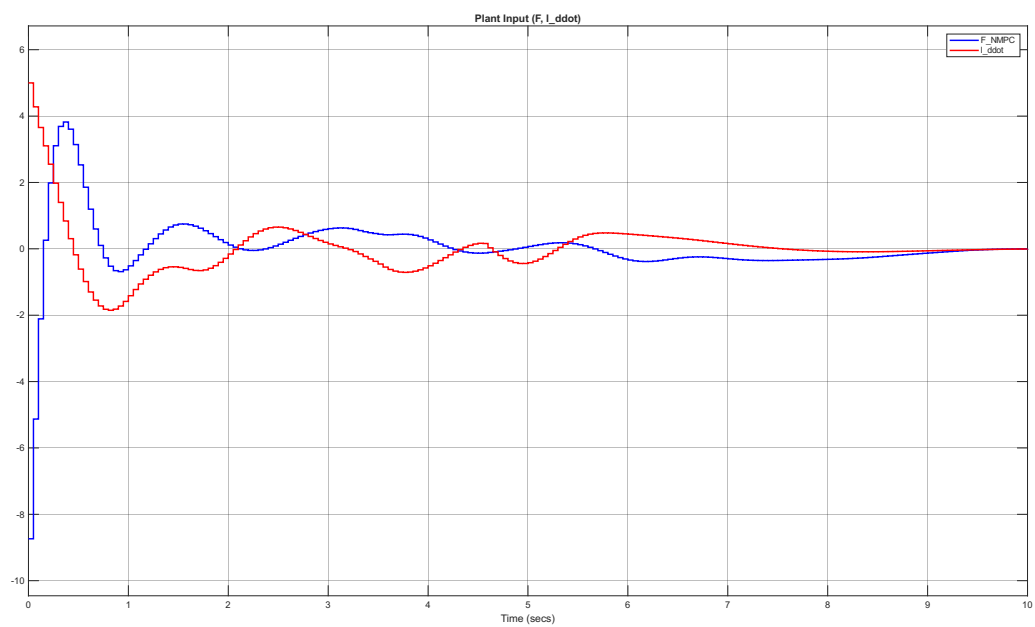
شکل ۱۷.۲ سیگنال‌های کنترلی اعمال شده به سیستم برای جابجایی ۵ متر
