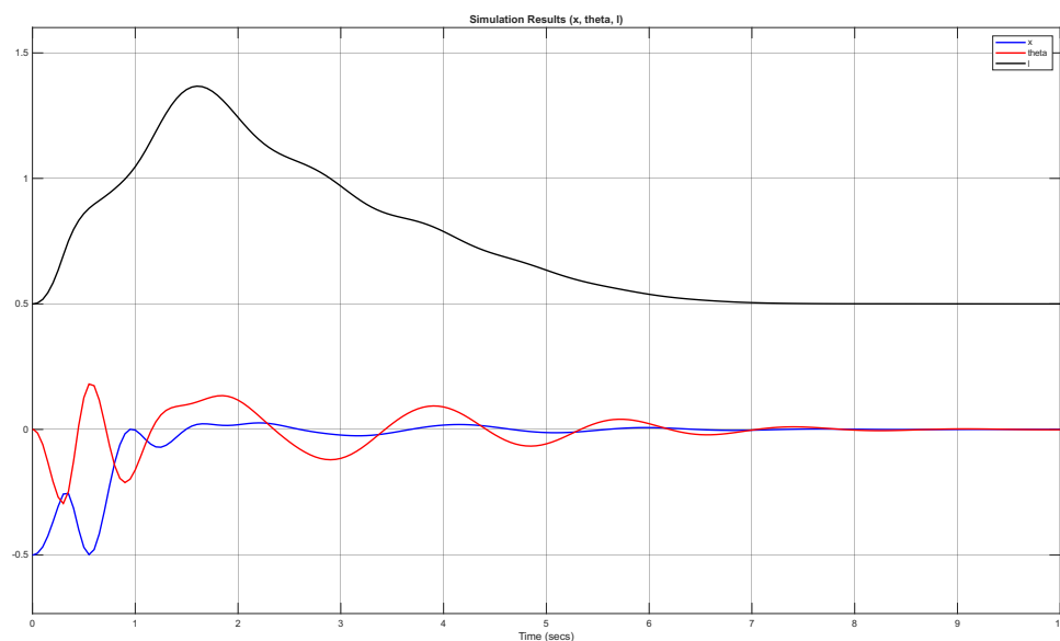
شکل ۱۵.۳ پاسخ زمانی موقعیت کالسکه، زاویه نوسان و طول کابل تحت ورودی پله
