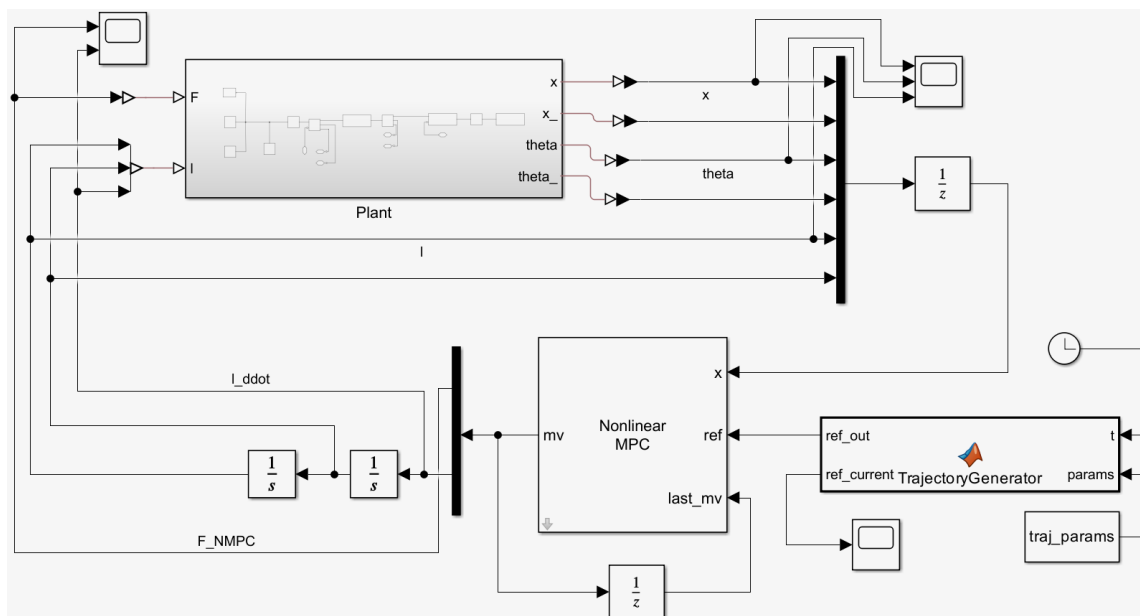
شکل ۱۶.۳ معماری نهایی حلقه کنترل پیش بین یکپارچه فاقد فیدفوروارد خارجی
