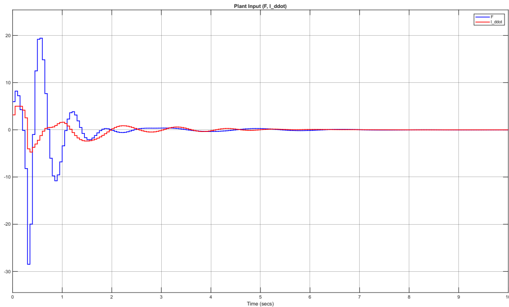
شکل ۱۳.۳ پروفایل سیگنال‌های کنترلی پایه؛ تلاش تهاجمی بهینه‌ساز برای غلبه بر خطای پله ضمن رعایت قیود فیزیکی عملگرها.
