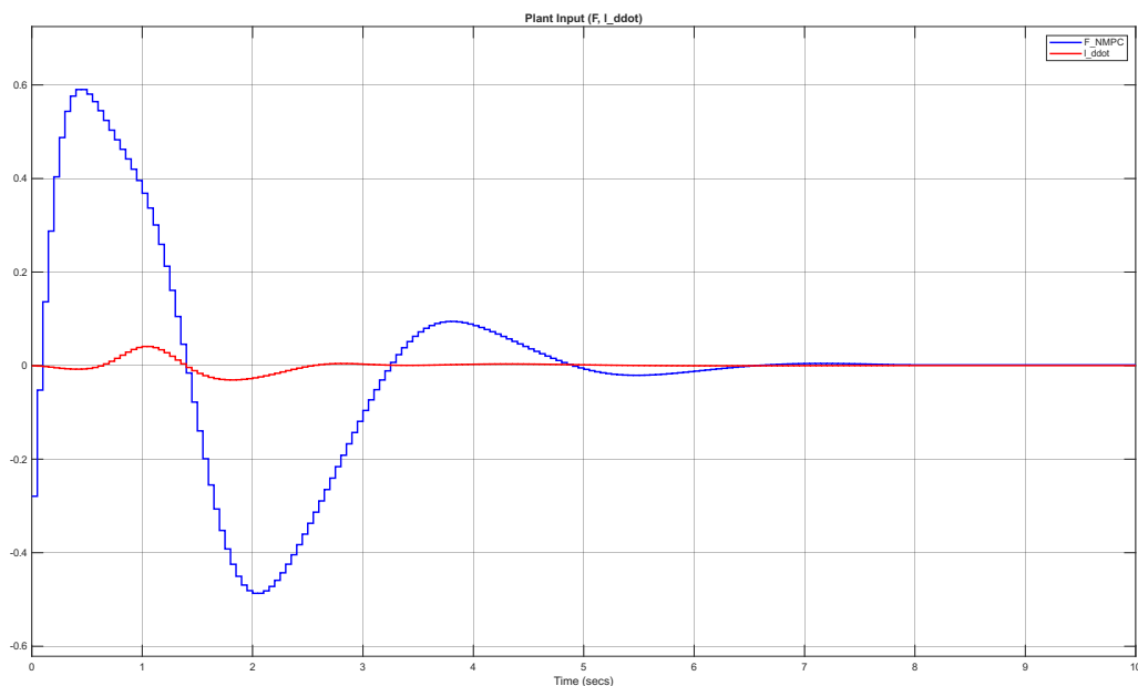
شکل ۱۸.۳ سیگنال‌های کنترلی بهینه‌سازی شده برای جابجایی ۰/۵ متر
