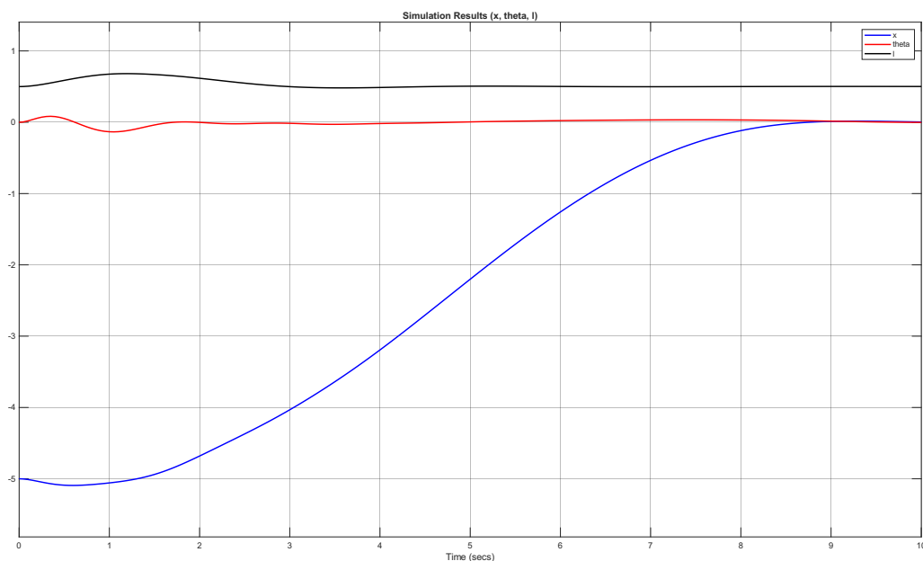
شکل ۱۹.۳ ردیابی دقیق و حذف کامل نوسانات پسماند در جابجایی ۵ متر
