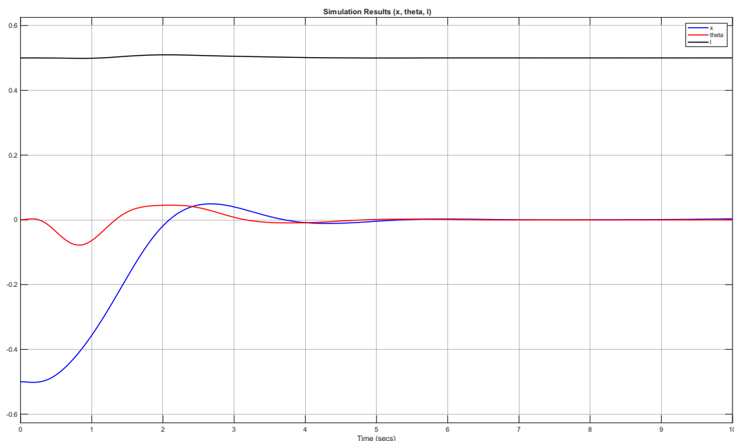
شکل ۱۷.۳ پاسخ زمانی موقعیت، زاویه و طول کابل در معماری یکپارچه (جابجایی ۵/۰ متر)
