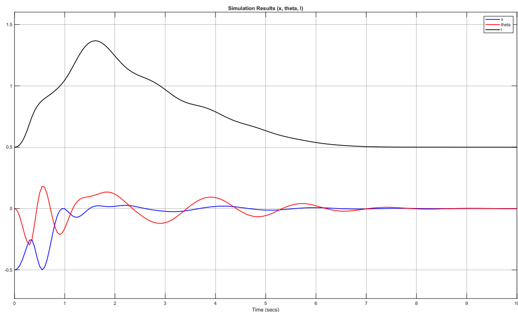
شکل ۱۲.۳ پاسخ زمانی متغیرهای حالت تحت هدایت NMPC؛ مانور رفت و برگشتی کالسکه و میرایی فعال از طریق افزایش طول کابل.
