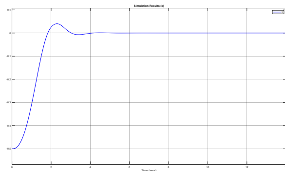
شکل ۷.۳ ردیابی موقعیت کالسکه در جابجایی ۰/۵ متر
