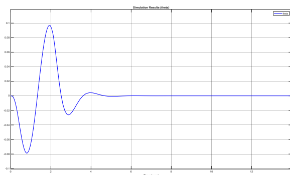
شکل ۸.۳ زاویه نوسان آونگ در جابجایی ۰/۵ متر
