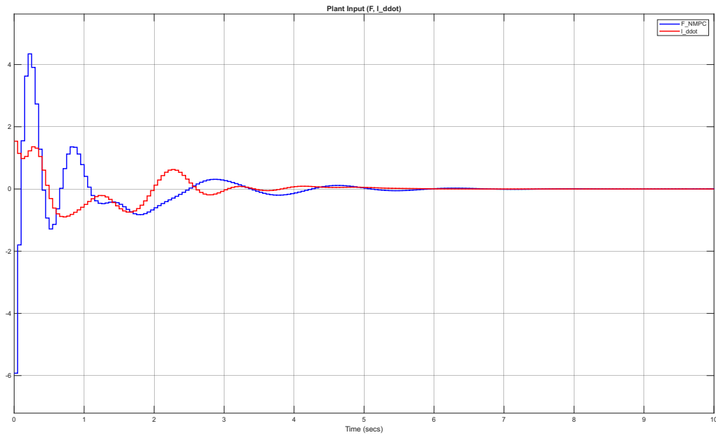
شکل ۱۸.۳ سیگنال‌های کنترلی بهینه‌سازی شده برای جابجایی ۵/۰ متر
