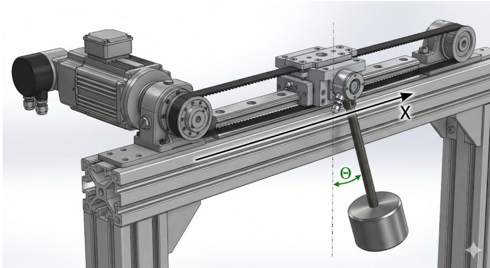
شکل ۲.۱ شماتیک طراحی و پروتوتایپ آزمایشگاهی سیستم جثقیل سقفی با مفصل کشویی متغیر (تغییر طول کابل).
