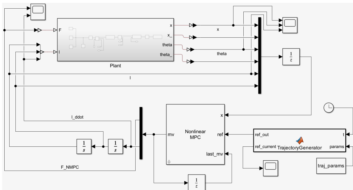
شکل ۲۵.۳ معماری نهایی حلقه کنترل پیش بین یکپارچه فاقد فیدفوروارد خارجی
