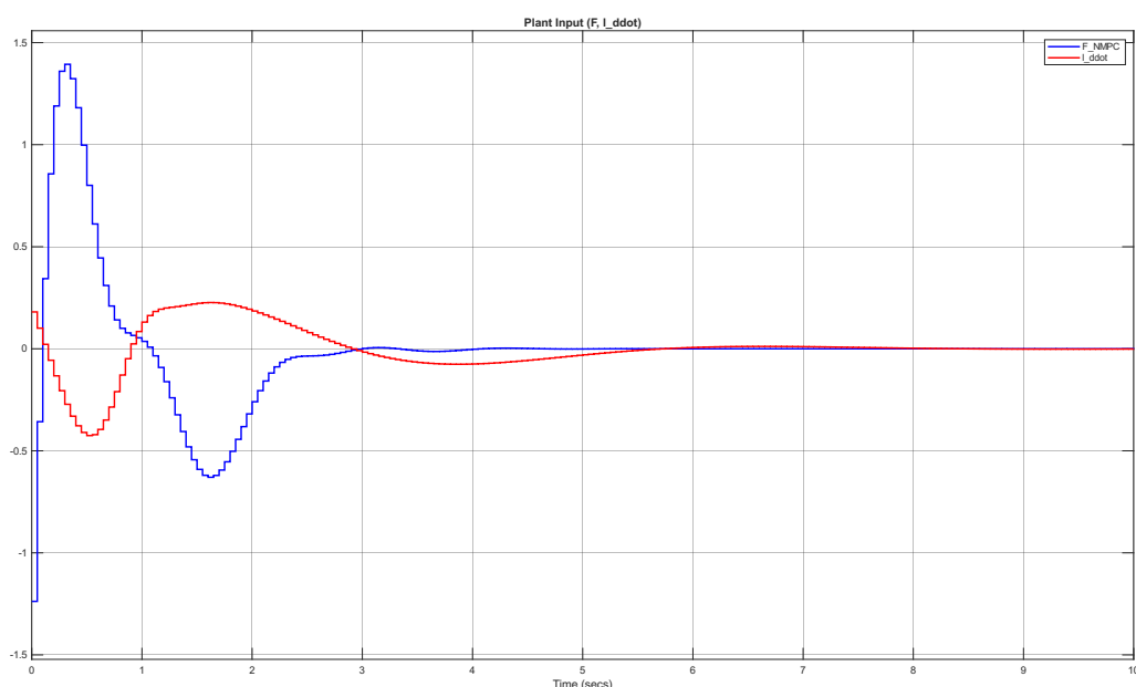
شکل ۲۷.۳ سیگنال‌های کنترلی بهینه‌سازی شده برای جابجایی ۰/۵ متر
