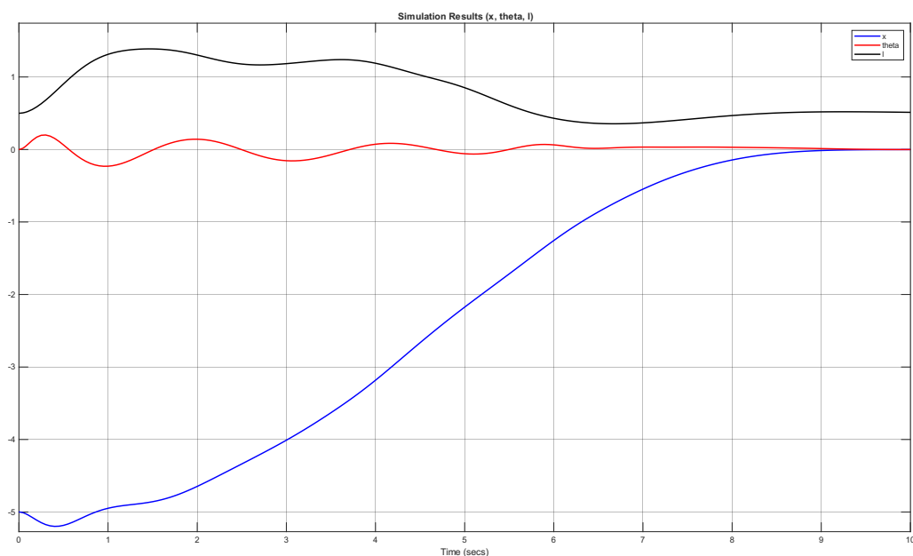
شکل ۲۸.۳ ردیابی دقیق و حذف کامل نوسانات پسماند در جابجایی ۵ متر
