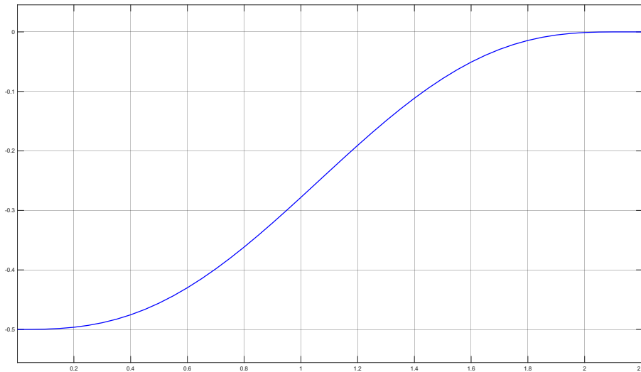
شکل ۱۵.۳ پروفایل مسیر مرجع نرم تولید شده توسط برنامه‌ریز سینماتیکی
