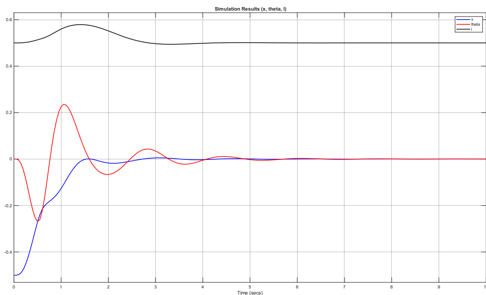
شکل ۲۲.۳ پاسخ زمانی موقعیت کالسکه، زاویه نوسان و طول کابل تحت ورودی پله
