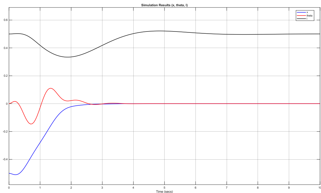
شکل ۱۷.۳ پاسخ زمانی موقعیت، زاویه و طول کابل در معماری یکپارچه (جابجایی ۰/۵ متر)
