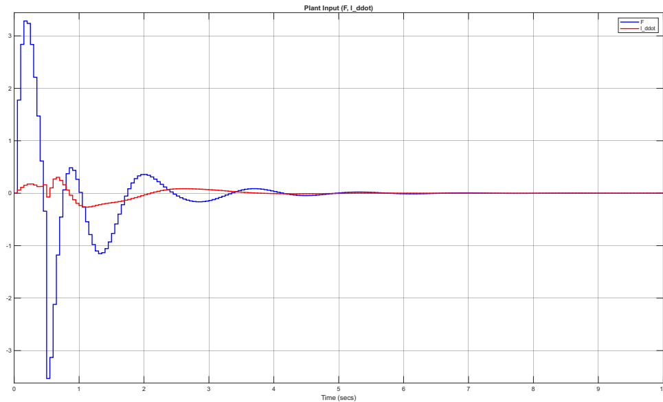
شکل ۲۳.۳ سیگنال‌های کنترلی پایه: نیروی کالسکه ( F ) و شتاب تغییر طول کابل ( \ddot{I} )
