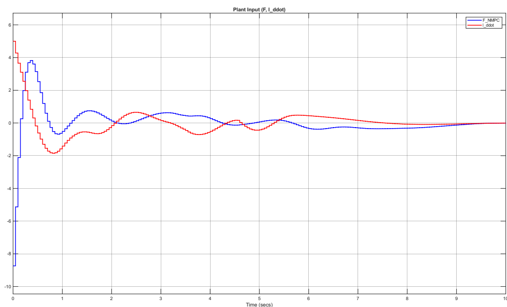
شکل ۲۹.۳ مدیریت ایمن عملگرها در شبیه‌سازی جابجایی بلندبرد ۵ متری
