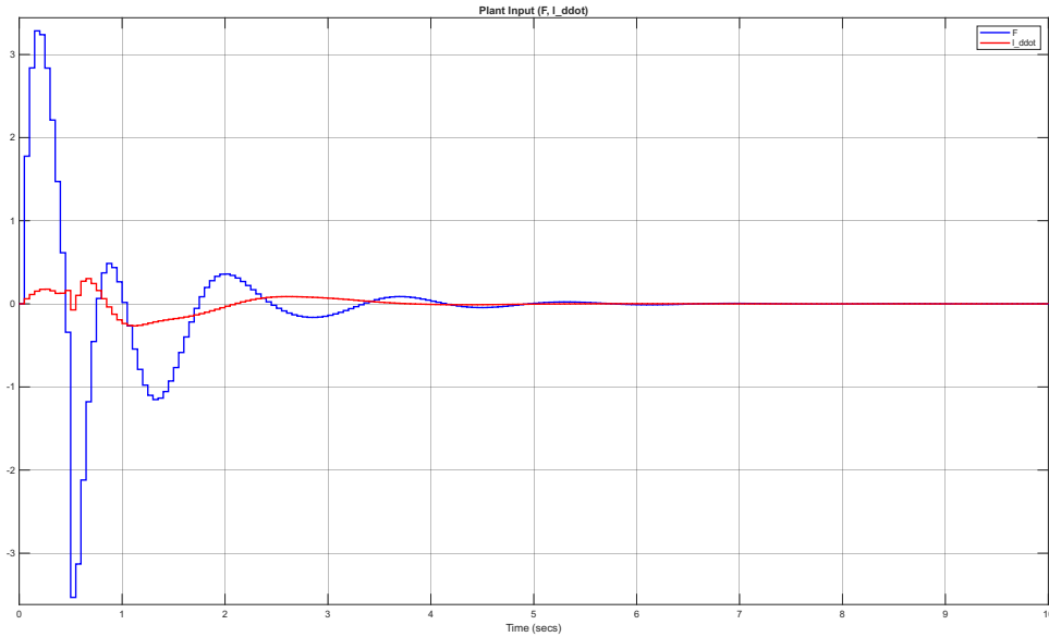
شکل ۱۴.۳ سیگنال‌های کنترلی پایه: نیروی کالسکه ( F ) و شتاب تغییر طول کابل ( \ddot{I} )
