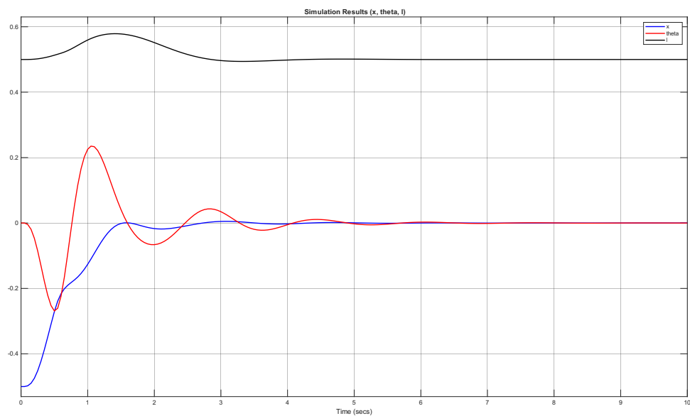
شکل ۱۳.۳ پاسخ زمانی موقعیت کالسکه، زاویه نوسان و طول کابل تحت ورودی پله
