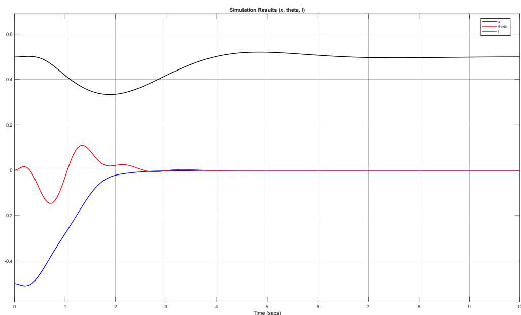
شکل ۲۶.۳ پاسخ زمانی موقعیت، زاویه و طول کابل در معماری یکپارچه (جابجایی ۰/۵ متر)
