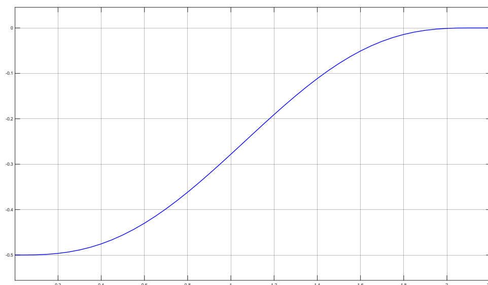
شکل ۵.۲ نمونه‌ای از پروفایل مسیر مرجع نرم (S-Curve) تولید شده توسط برنامه‌ریز سینماتیکی برای جابجایی ۰/۵ متر.
