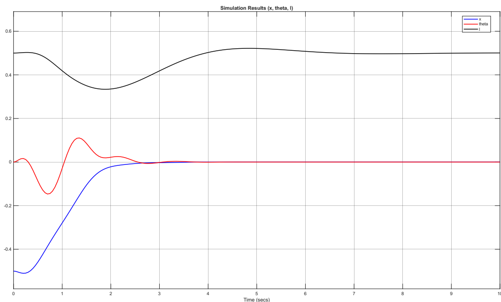
شکل ۲۷.۳ پاسخ زمانی موقعیت، زاویه و طول کابل در معماری یکپارچه (جابجایی ۰/۵ متر)
