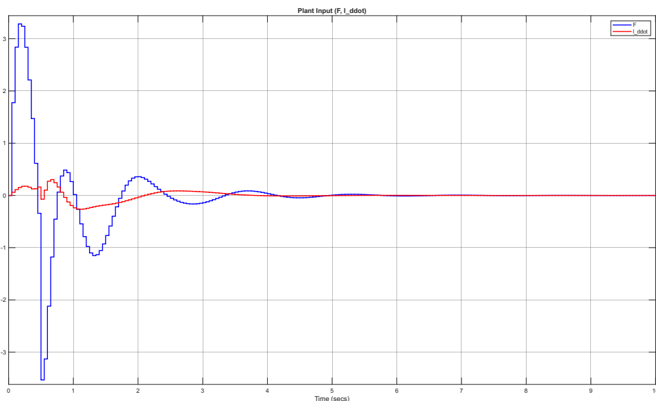
شکل ۲۴.۳ سیگنال‌های کنترلی پایه: نیروی کالسکه ( F ) و شتاب تغییر طول کابل ( \ddot{l} )
