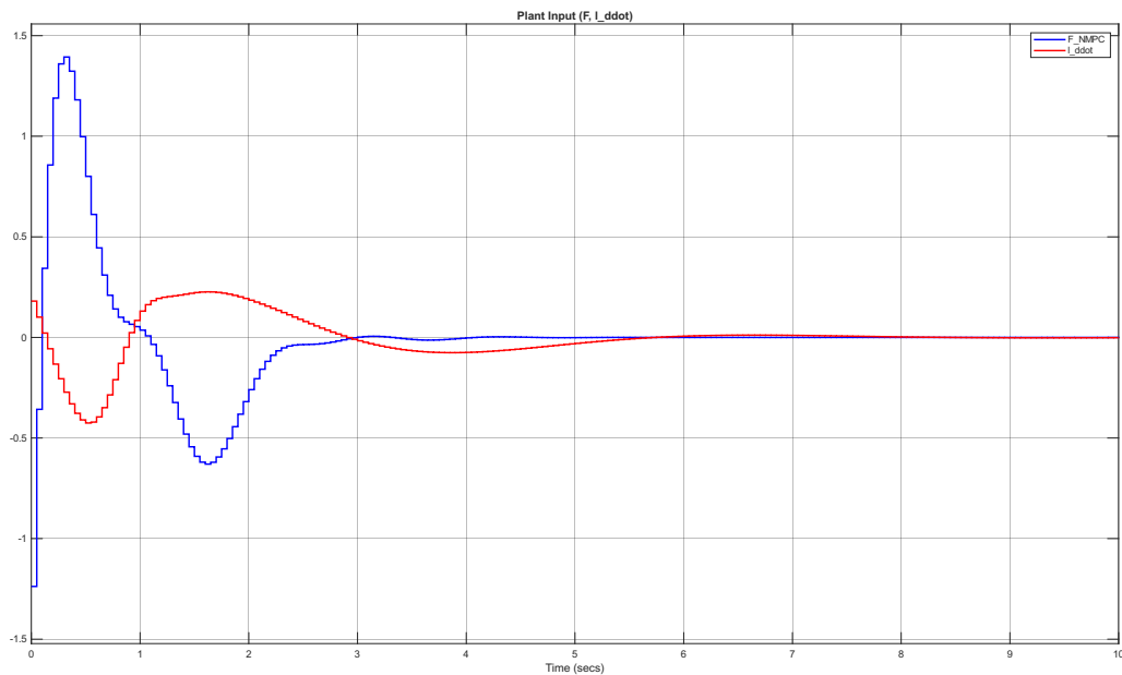
شکل ۲۸.۳ سیگنال‌های کنترلی بهینه‌سازی شده برای جابجایی ۰/۵ متر
