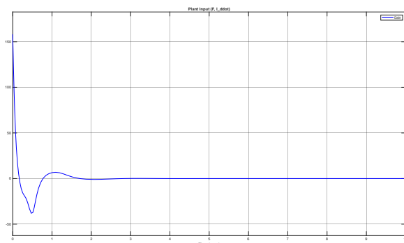
شکل ۴.۳ نیروی کنترلی در جابجایی ۵ متر (اشباع شدید عملگر)
