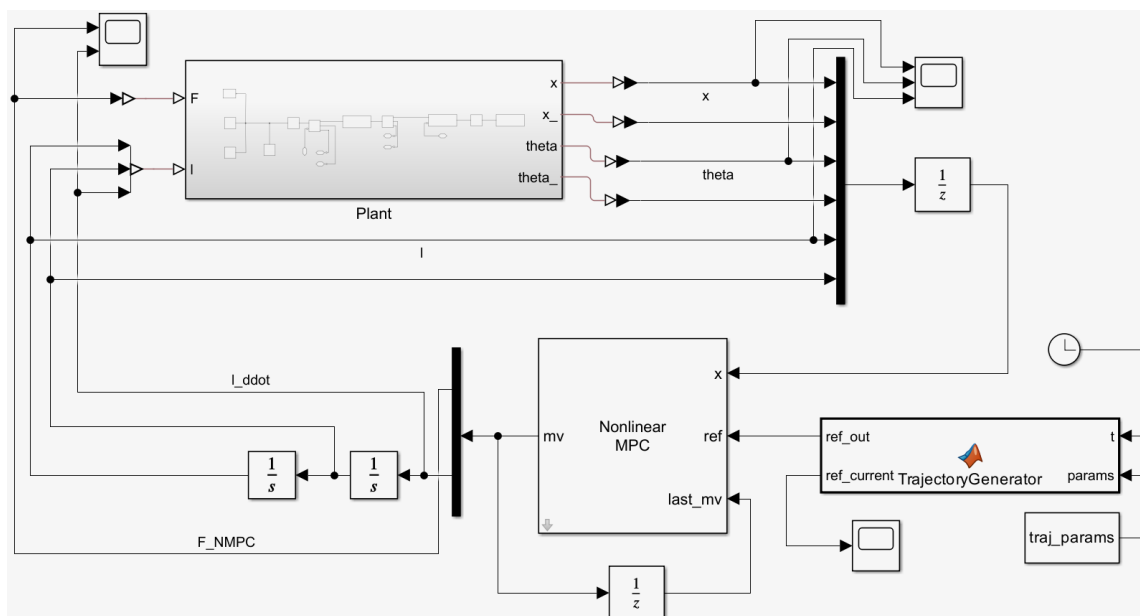
شکل ۱۸.۳ معماری نهایی حلقه کنترل پیش‌بین یکپارچه فاقد فیدفوروارد خارجی
