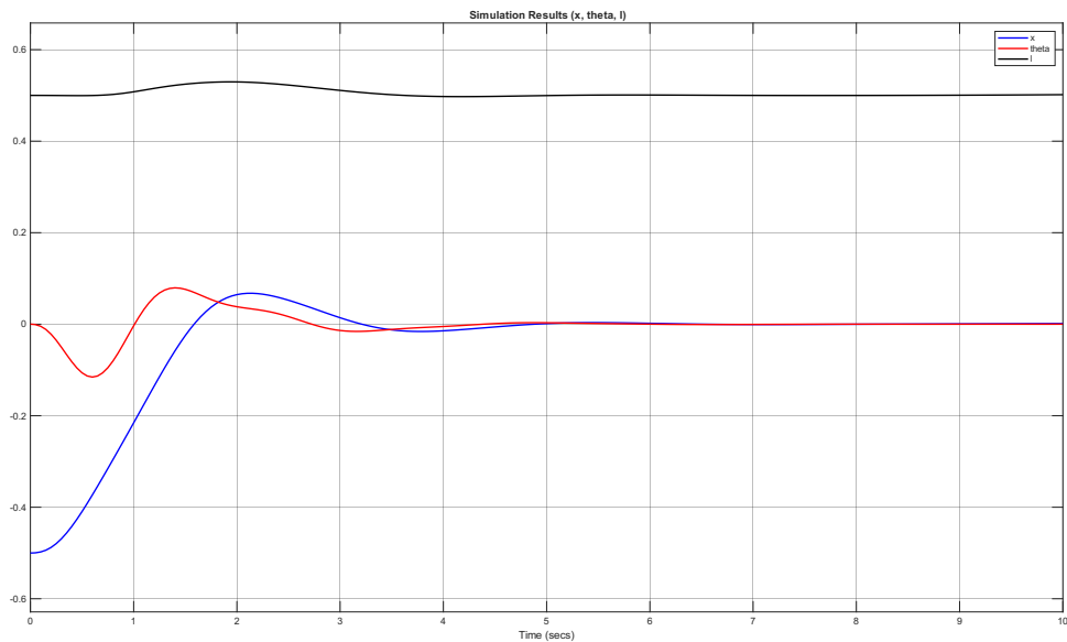
شکل ۱۷.۳ پاسخ زمانی موقعیت کالسکه، زاویه نوسان و طول کابل تحت ورودی پله
