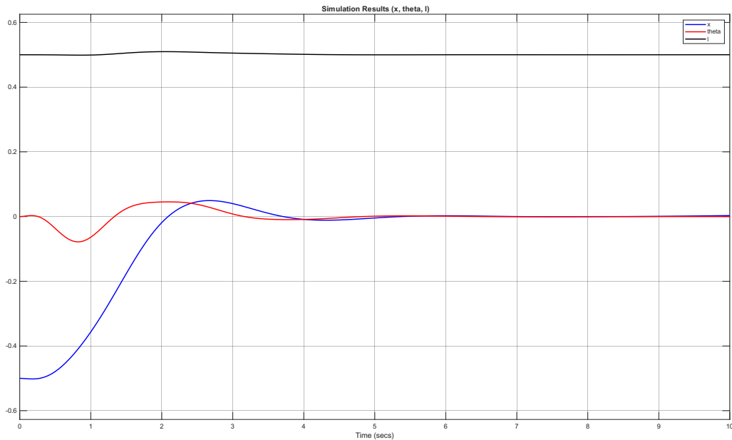
شکل ۱۹.۳ پاسخ زمانی موقعیت، زاویه و طول کابل در معماری یکپارچه (جابجایی ۰/۵ متر)
