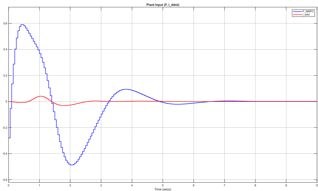
شکل ۲۰.۳ سیگنال‌های کنترلی بهینه‌سازی شده برای جابجایی ۰/۵ متر
