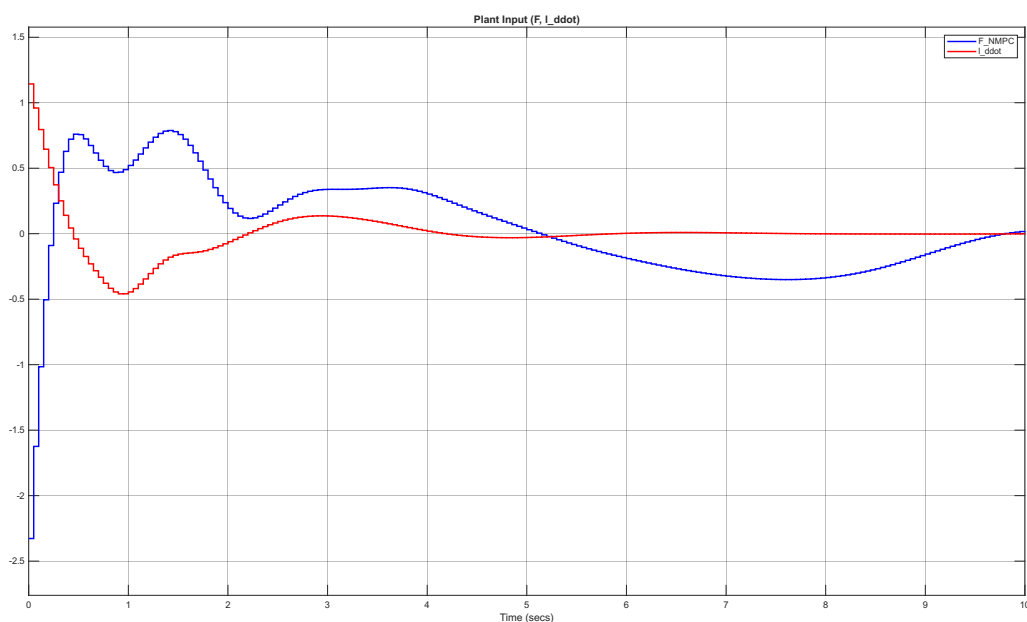
شکل ۲۲.۳ مدیریت ایمن عملگرها در شبیه‌سازی جابجایی بلندبرد ۵ متری
