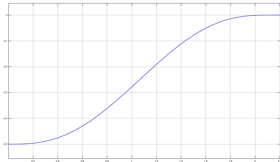
شکل ۶.۲ نمونه‌ای از پروفایل مسیر مرجع نرم (S-Curve) تولید شده توسط برنامه‌ریز سینماتیکی برای جابجایی ۰/۵ متر.
