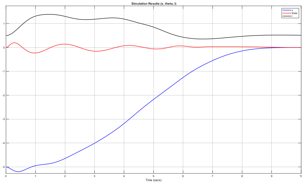
شکل ۲۹.۳ ردیابی دقیق و حذف کامل نوسانات پسماند در جابجایی ۵ متر
