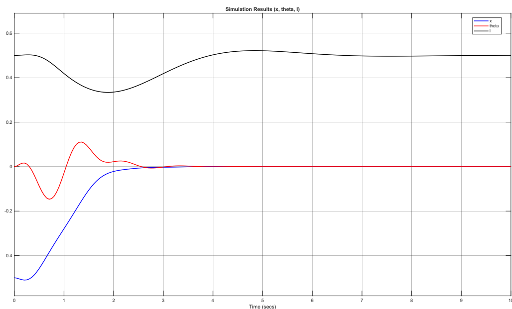
شکل ۲۷.۳ پاسخ زمانی موقعیت، زاویه و طول کابل در معماری یکپارچه (جابجایی ۵/۰ متر)
