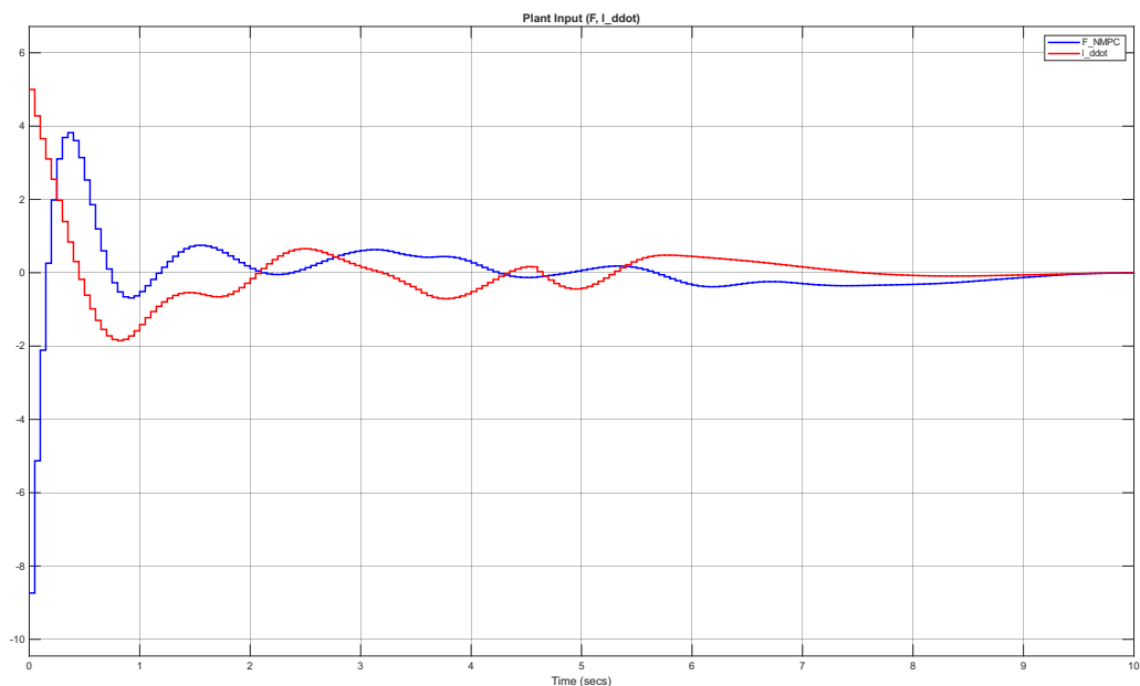
شکل ۲۱.۳ مدیریت ایمن عملگرها در شبیه‌سازی جابجایی بلندبرد ۵ متری
