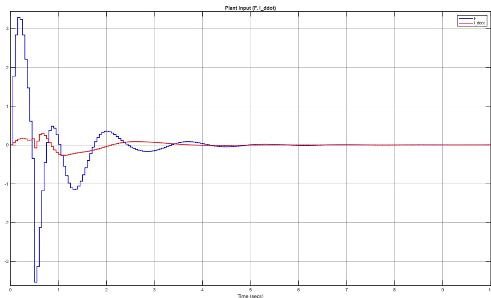
شکل ۱۵.۳ سیگنال‌های کنترلی پایه: نیروی کالسکه ( F ) و شتاب تغییر طول کابل ( \ddot{l} )
