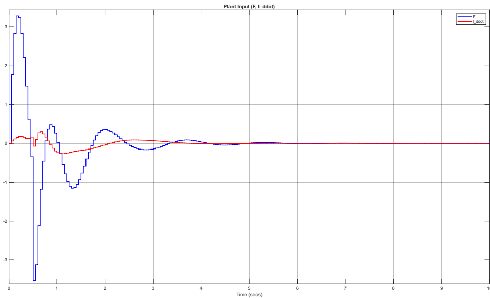
شکل ۲۴.۳ سیگنال‌های کنترلی پایه: نیروی کالسکه ( F ) و شتاب تغییر طول کابل ( \ddot{I} )
