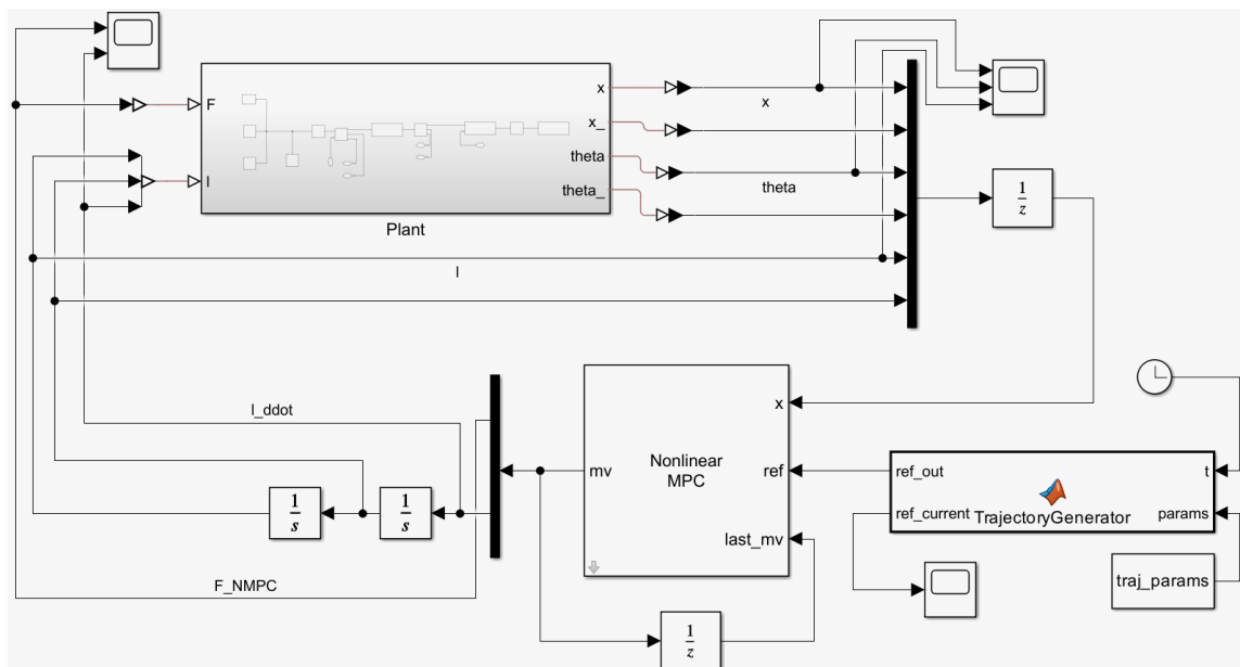
شکل ۱۷.۳ معماری نهایی حلقه کنترل پیش بین یکپارچه فاقد فیدفوروارد خارجی
