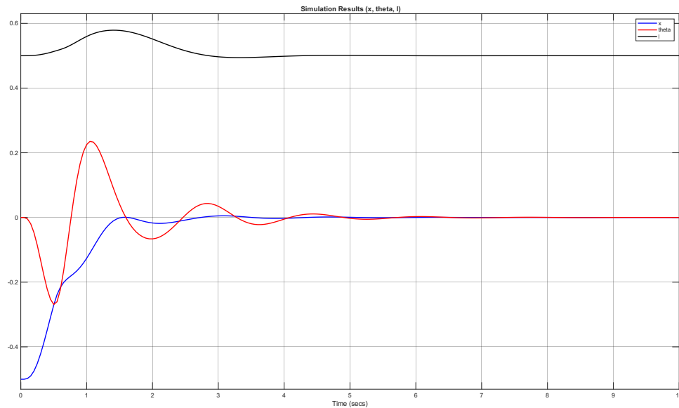
شکل ۲۳.۳ پاسخ زمانی موقعیت کالسکه، زاویه نوسان و طول کابل تحت ورودی پله
