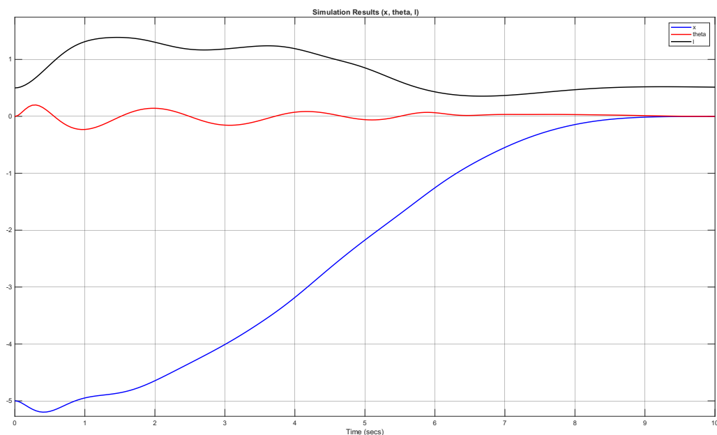
شکل ۲۰.۳ ردیابی دقیق و حذف کامل نوسانات پسماند در جابجایی ۵ متر
