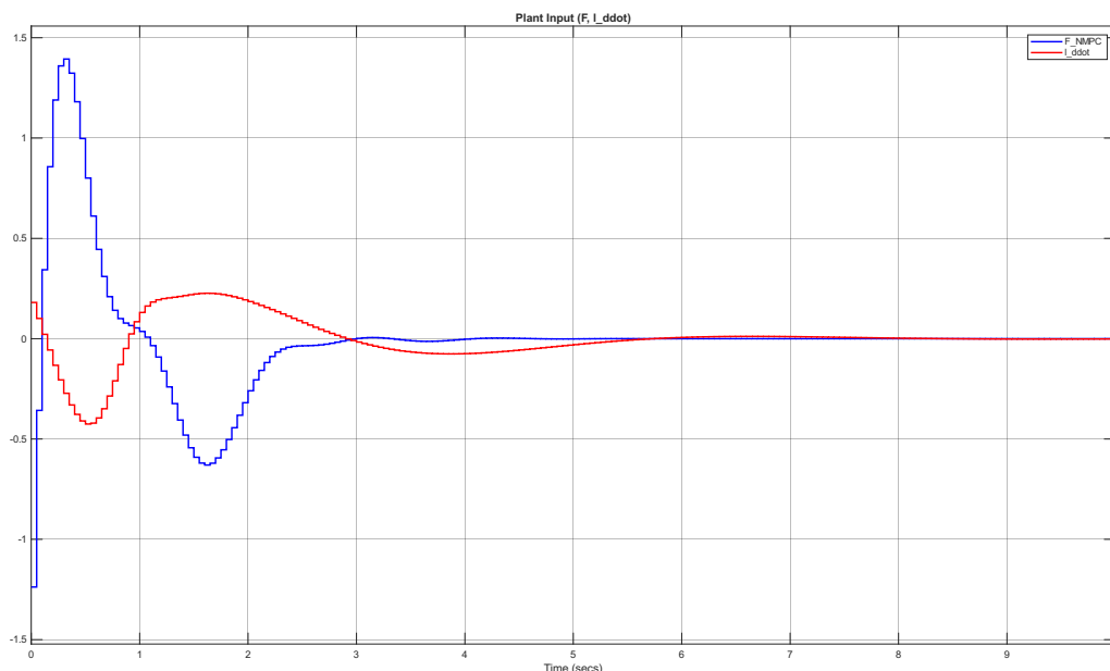
شکل ۲۸.۳ سیگنال‌های کنترلی بهینه‌سازی شده برای جابجایی ۵/۰ متر
