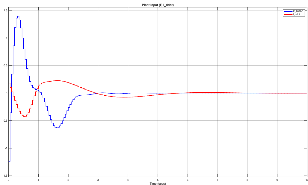
شکل ۱۹.۳ سیگنال‌های کنترلی بهینه‌سازی شده برای جابجایی ۰/۵ متر
