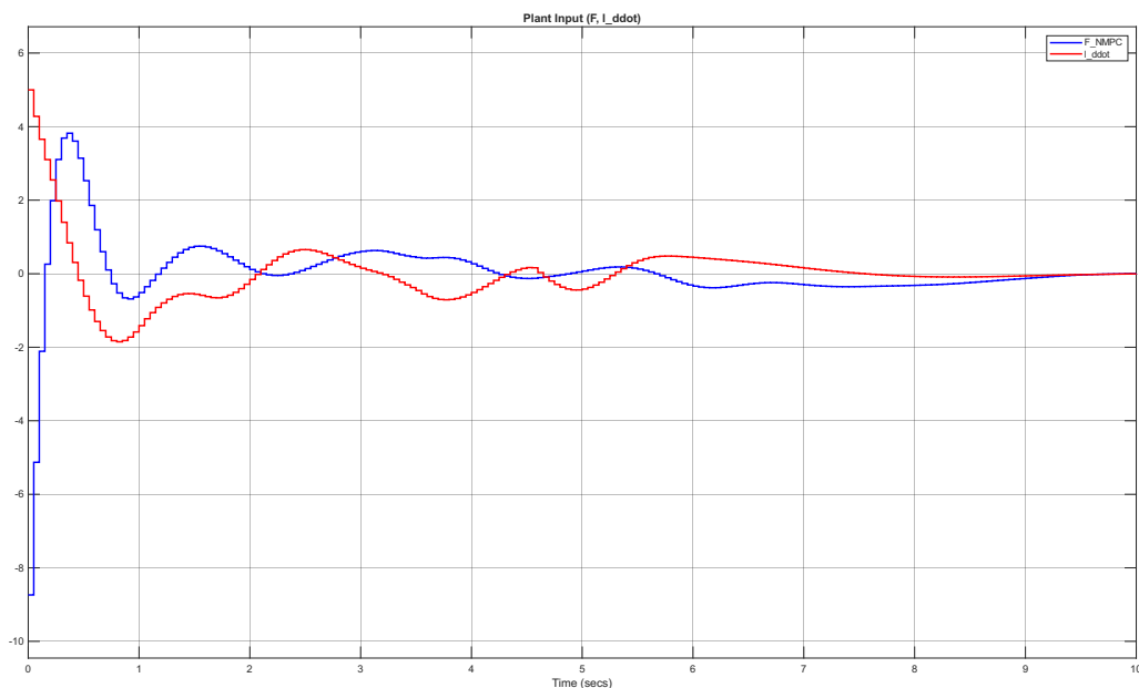
شکل ۳۰.۳ مدیریت ایمن عملگرها در شبیه‌سازی جابجایی بلندبرد ۵ متری
