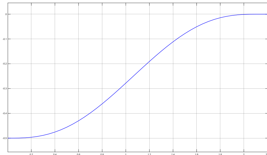
شکل ۲۵.۳ پروفایل مسیر مرجع نرم تولید شده توسط برنامه‌ریز سینماتیکی
