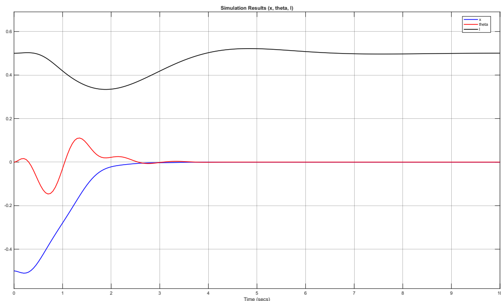
شکل ۱۸.۳ پاسخ زمانی موقعیت، زاویه و طول کابل در معماری یکپارچه (جابجایی ۵/۰ متر)
