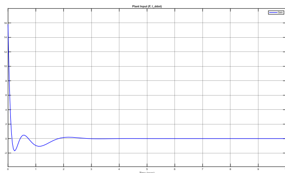
شکل ۴.۲ تلاش کنترلی (نیروی اعمالی کالسکه) برای جابجایی 0.5 متر
