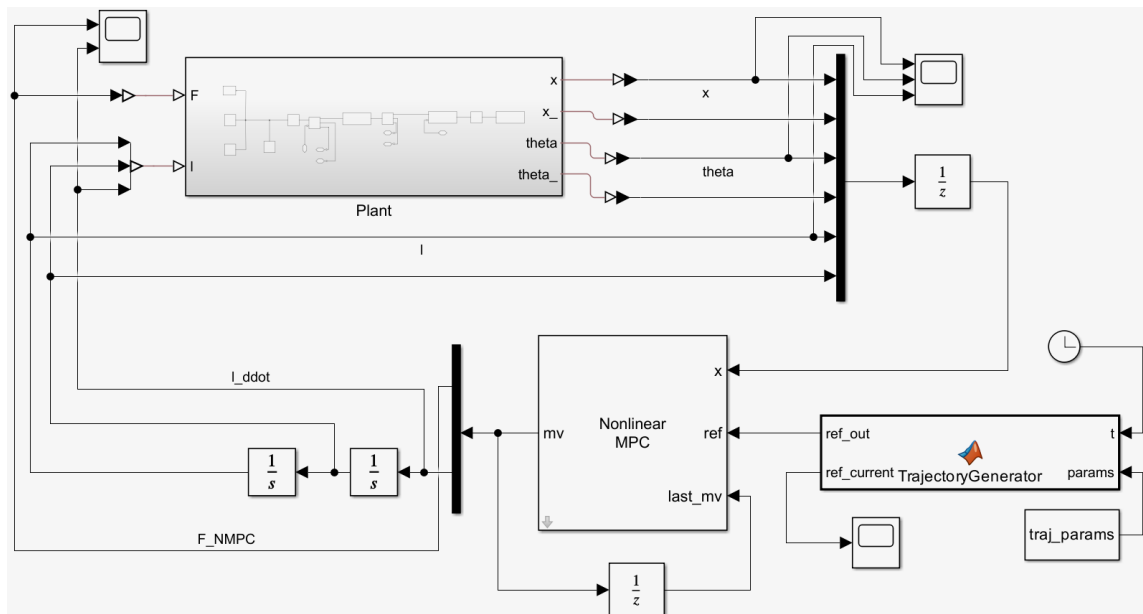
شکل ۱۲.۲ معماری نهایی حلقه کنترل پیش‌بین یکپارچه بدون فیدفوروارد خارجی
