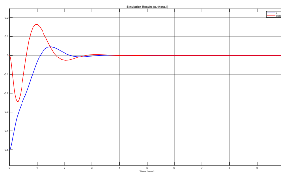
شکل ۳.۲ پاسخ زمانی موقعیت کالسکه و زاویه آونگ برای جابجایی 0.5 متر
