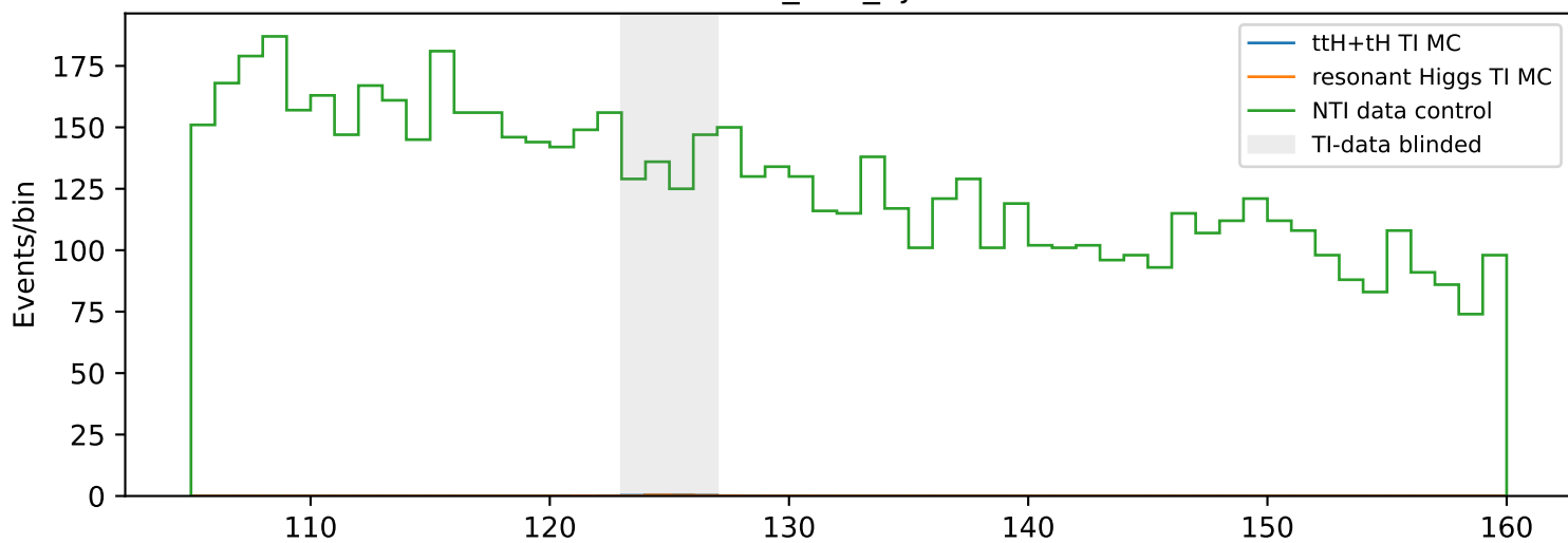
tH_had_4j2b
