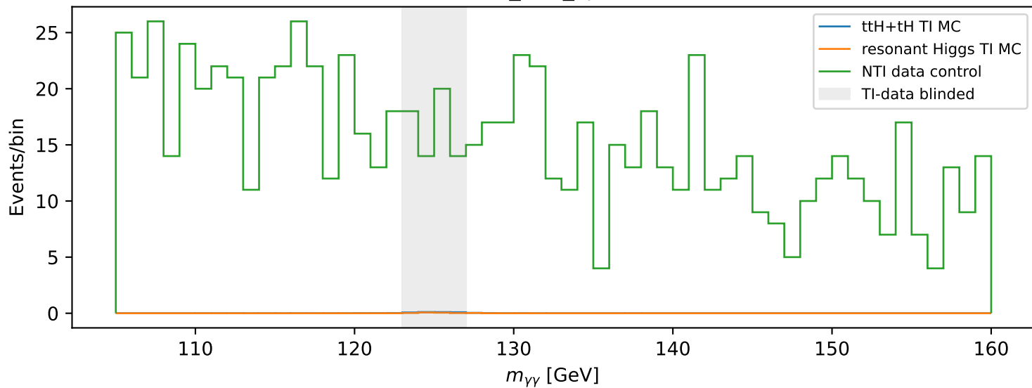
tH_had_4j2b
