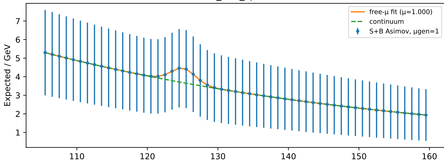
tH_had_4j2b
