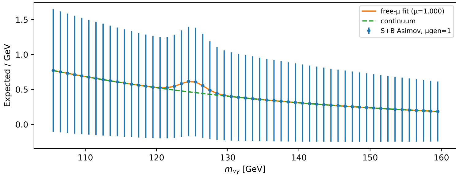
tH_had_4j2b
