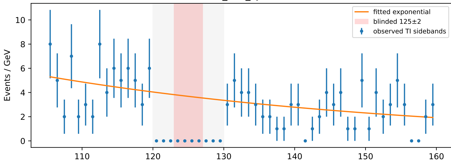
tH_had_4j2b
