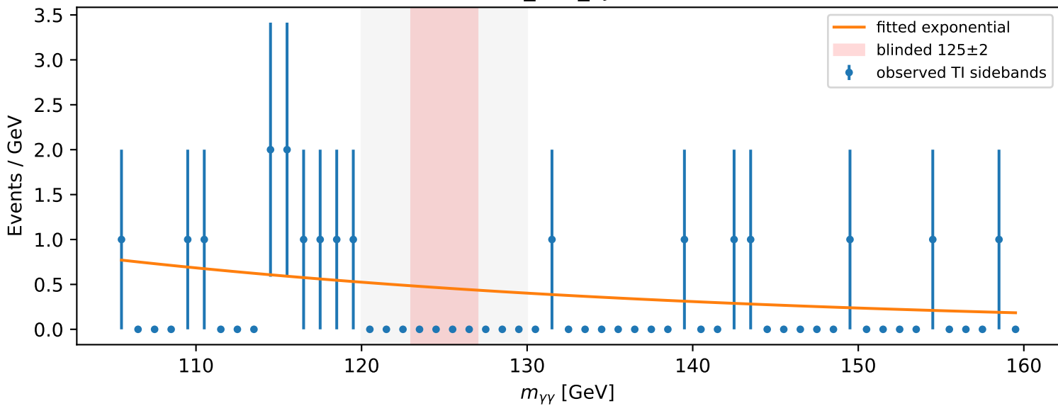
tH_had_4j2b
