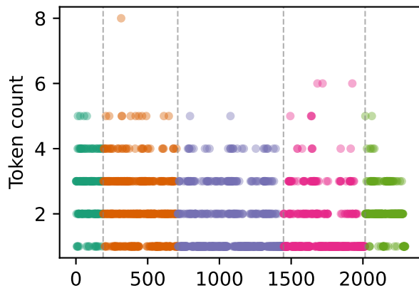
Gemma 4
