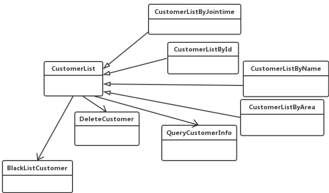
图 4.3 customer 模块简单类图
