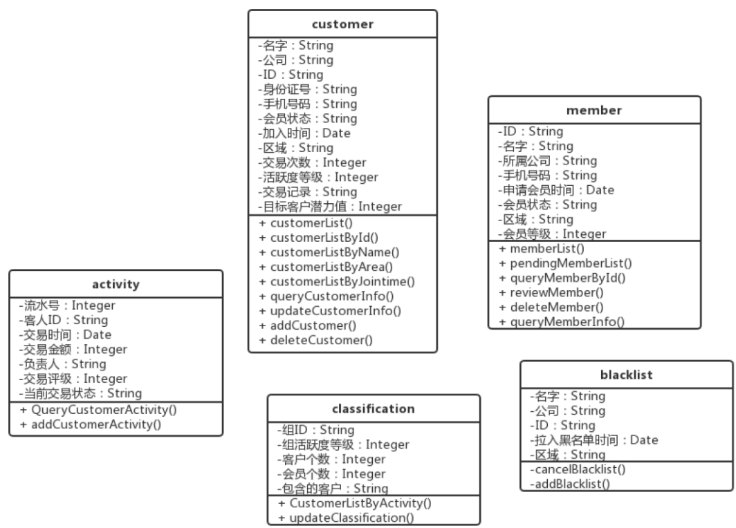
图 4.2 实体类图（包含属性和方法）
