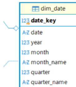
Hình 2.13 Lược đồ dim_date
