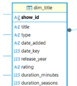
Hình 2.12 Lược đồ dim_title
