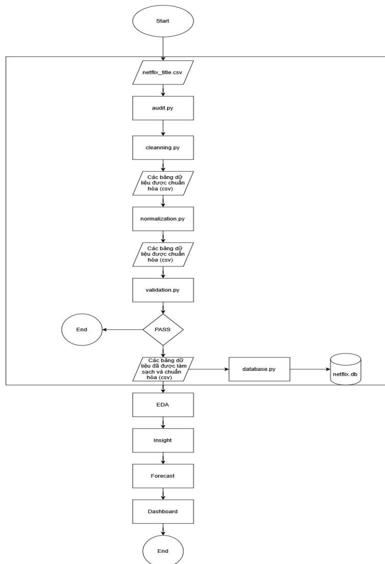
Hình 2.19 Pipeline xử lý dữ liệu của đề tài
