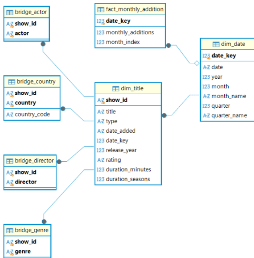
Hình 2.11 Mô hình dữ liệu gồm bảy bảng sau chuẩn hóa
