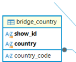
Hình 2.15 Lược đồ bridge_country
