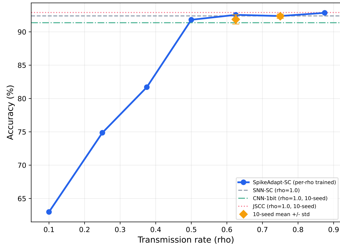
RESISC45: Clean (BER=0)
