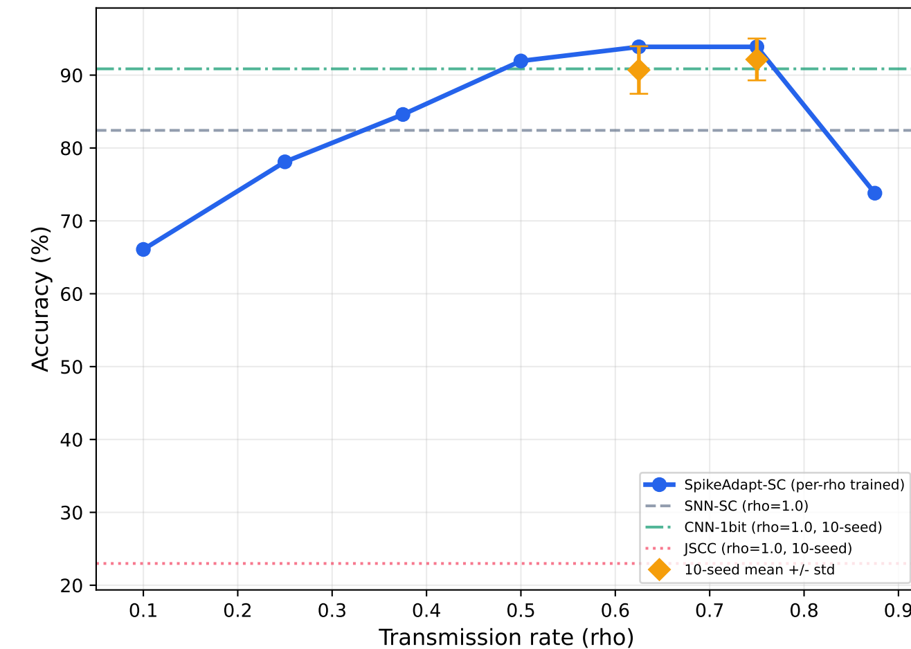
AID: BER=0.30
