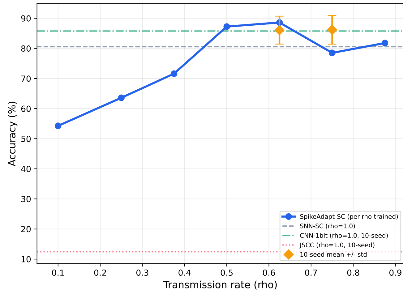
RESISC45: BER=0.30
