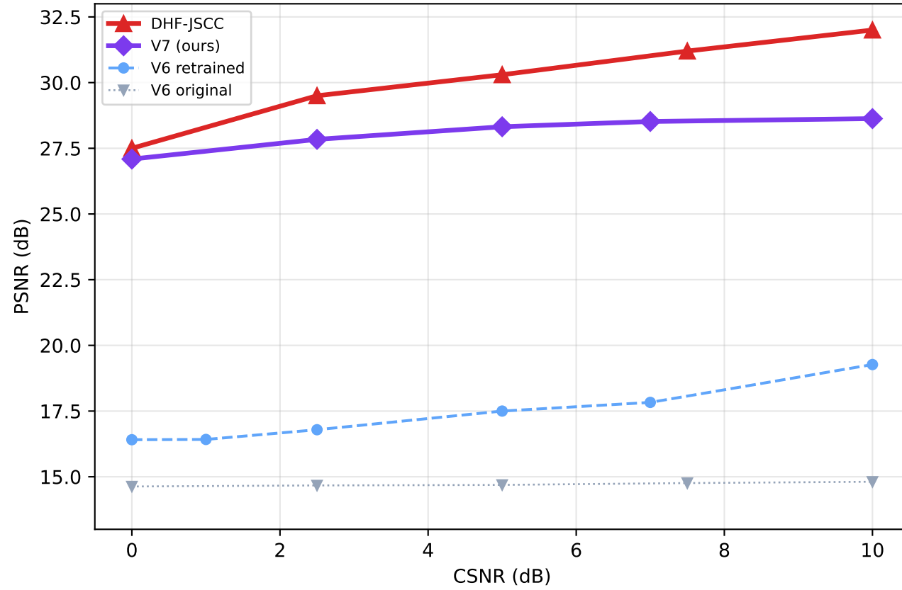
InStereo2K: AWGN (CBR=0.065)
