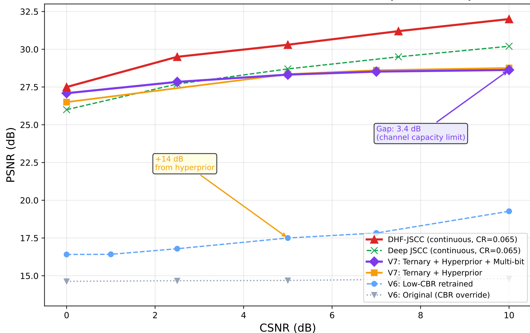
InStereo2K: Reconstruction PSNR vs CSNR (CBR=0.065)
