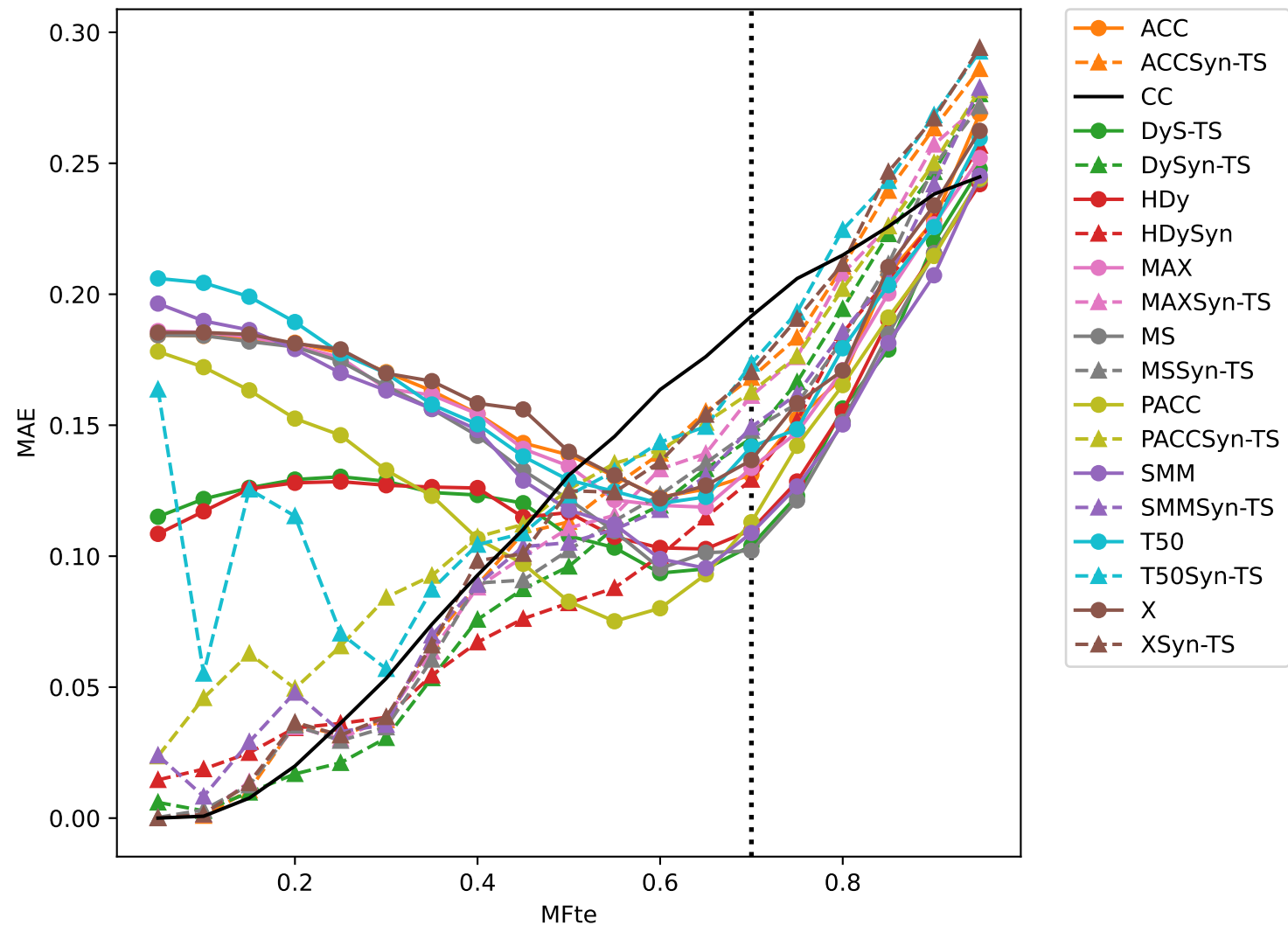
MAE vs MFte for MFtr = 0.7
