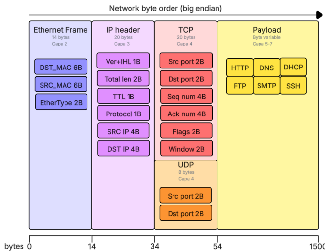
Figura 2. Estructura simplificada de un paquete de red.
