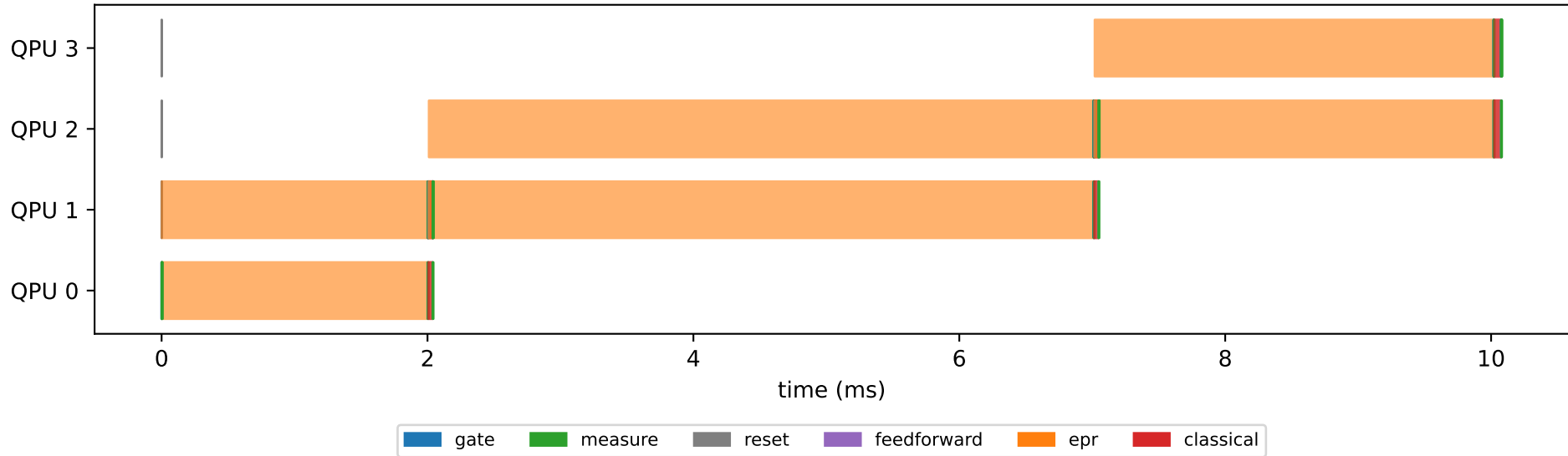
GHZ 12-qubit DQC timeline
