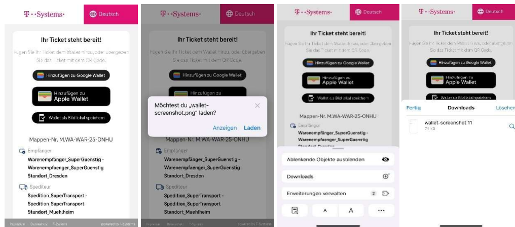
Abbildung 1: Download Wallet
