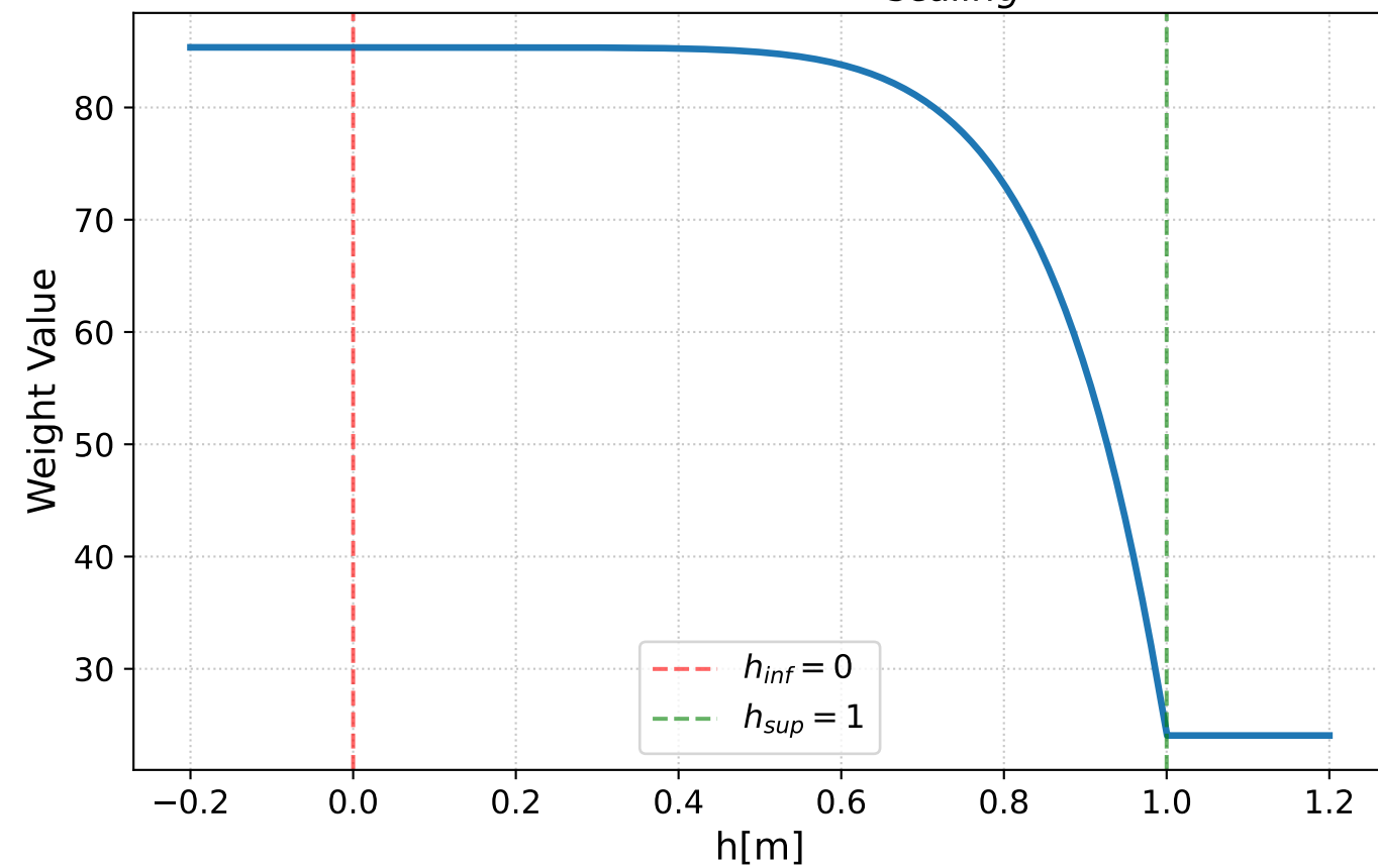
Parameter: \lambda_{scaling}
