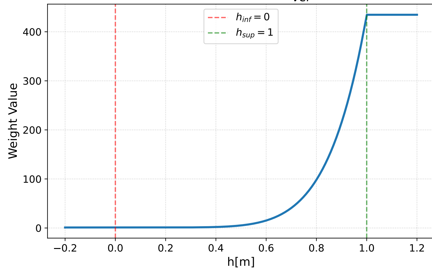
Parameter: \lambda_{scaling}
