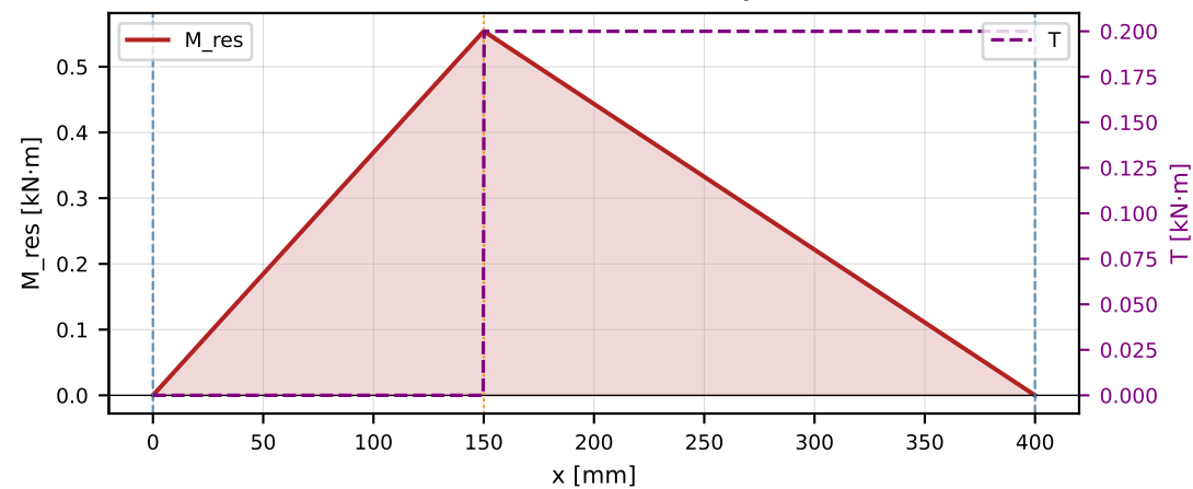
Momento resultante e torção
