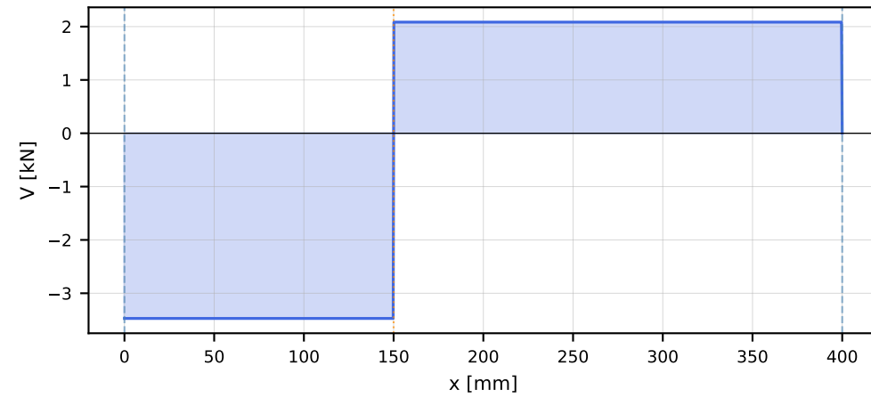
Esforço transversal — plano XZ
