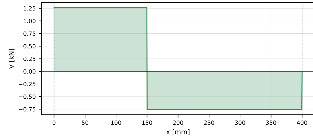
Esforço transversal — plano XY
