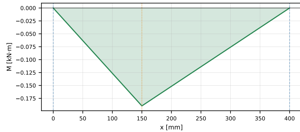
Momento fletor — plano XY
