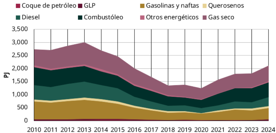
Figura 13. Figura 4.2 Evolución de producción de energía en refineries y despuntadoras por energético, 2010-2024
