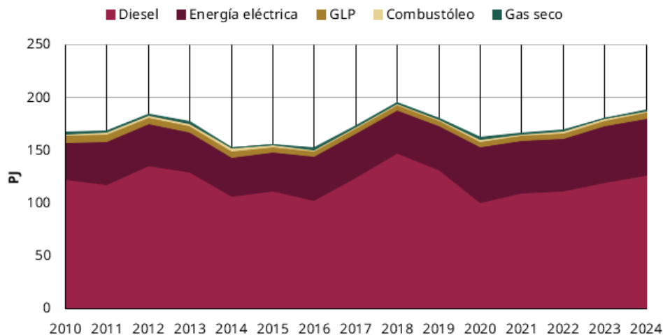
Figura 25. Figura 5.4 Evolución del consumo energético del sector agropecuario por energético, 2010-2024
