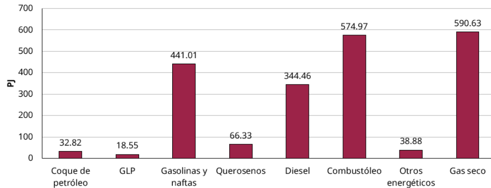
Figura 12. Figura 4.1 Composición de la transformación en refinerías y despuntadoras por energético, 2024
