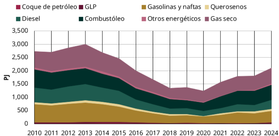
Figura 13. Figura 4.2 Evolución de producción de energía en refinerías y despuntadoras por energético, 2010-2024
