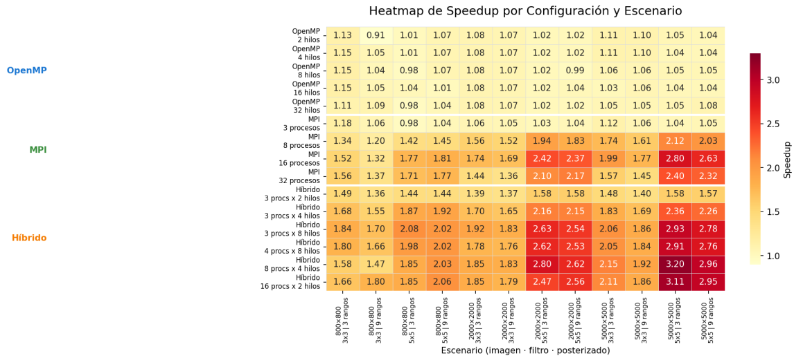
Figura 3.4: Heatmap de Speedup detallado por escenario y configuración en el cluster.
