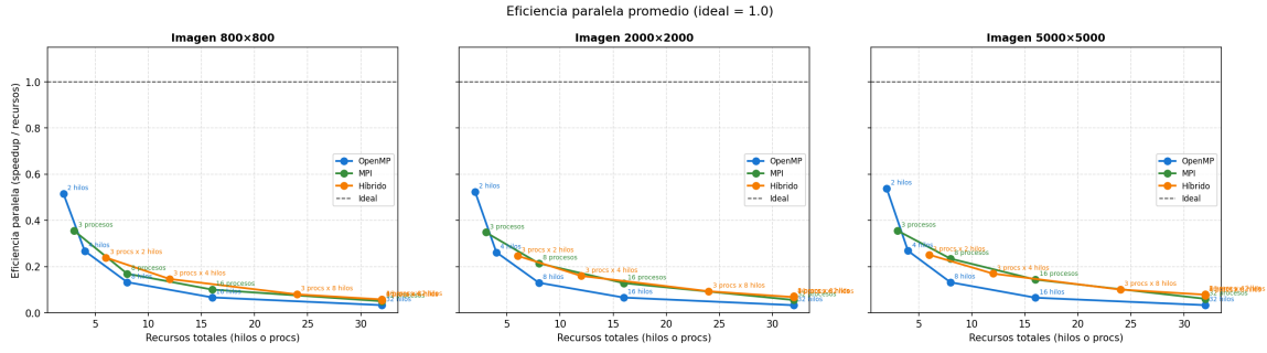
Figura 3.3: Eficiencia paralela promedio en Entorno cluster comparando OpenMP, MPI e Híbrido frente al comportamiento Ideal.
