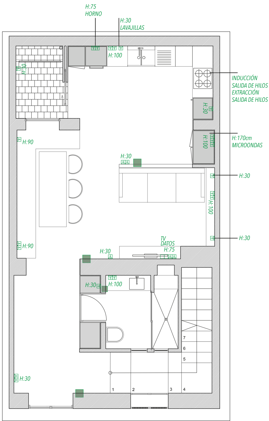
PLANTA BAJA
