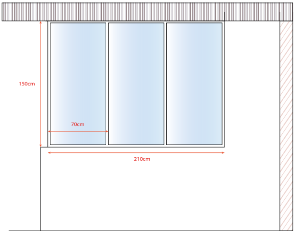
PB3 Estructura de cristales fijos
