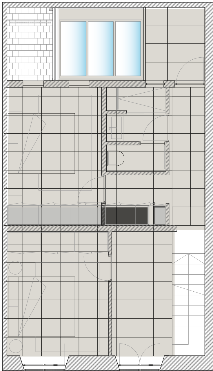
DESPIECE PLANTA PRIMERA
