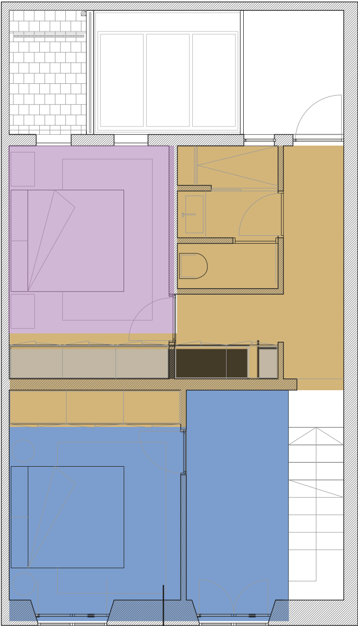
PLANTA PRIMERA
