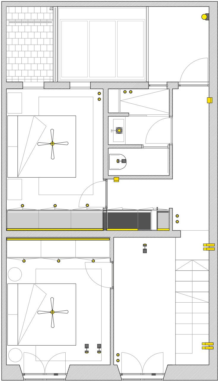
PLANTA PRIMERA
