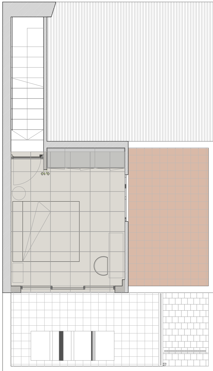
DESPIECE PLANTA BAJA
