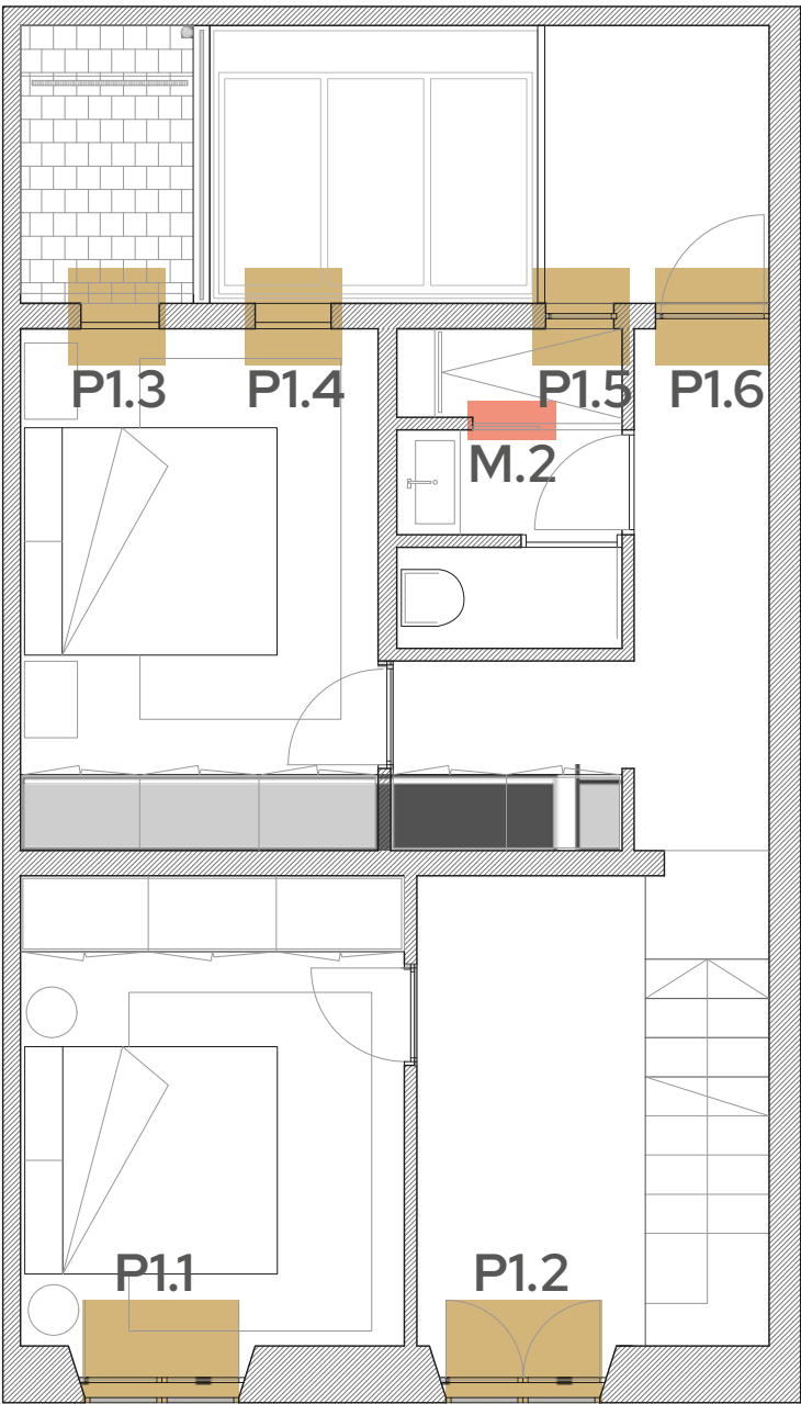
PLANTA PRIMERA
