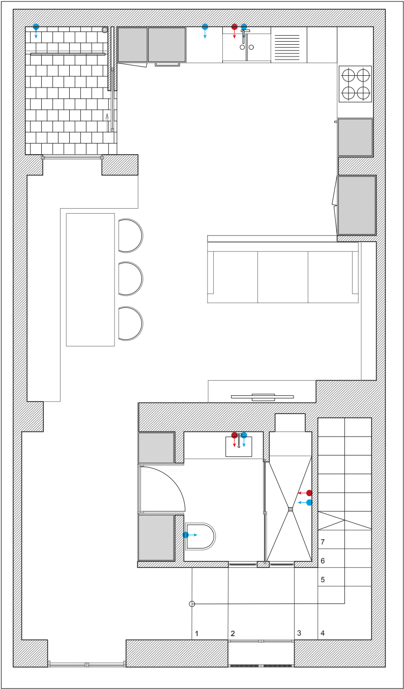
PLANTA BAJA
