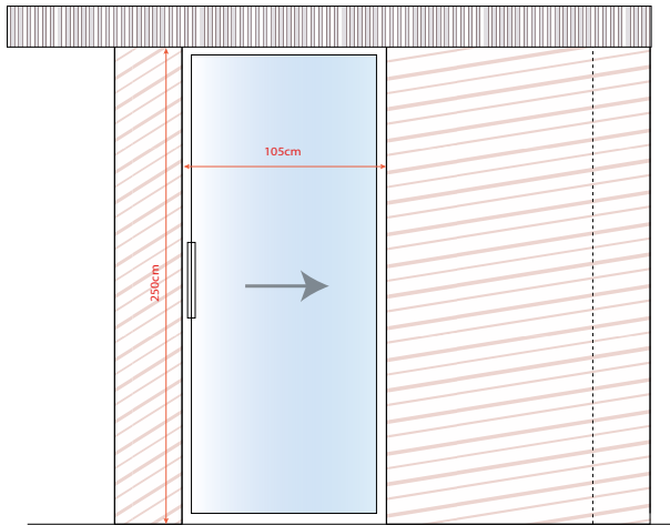
PB1 Puerta corredera entre muros
