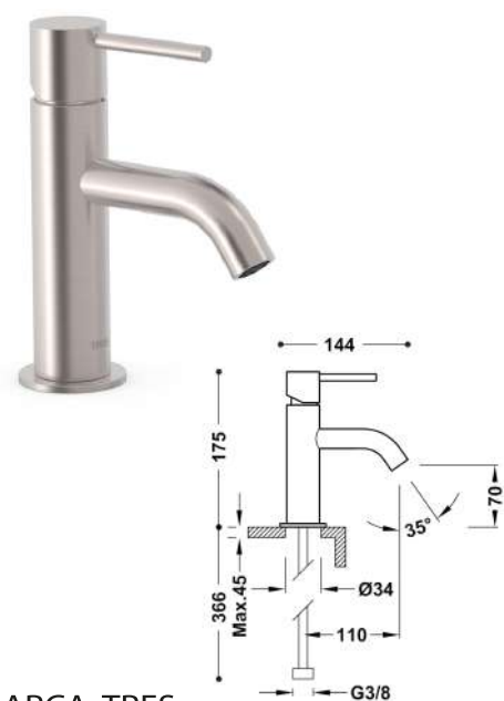
MARCA: TRES Ref. 26290301AC STUDY GRIFO MONOMANDO PARA LAVABO Acabado ACERO 1 UNIDAD
