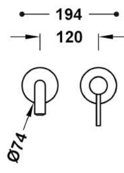
MARCA: TRES Ref. 26230021AC STUDY PIEZA VISTA PARA CUERPO EMPOTRADO DE LAVABO-26230021AC
