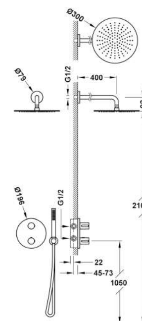
MARCA: TRES Ref. 26225004AC THERM-BOX KIT DE GRIFO TERMOSTÁTICO EMPOTRADO DE 2 VÍAS THERM-BOX PARA DUCHA-26225004AC Acabado ACERO 2 UNIDADES
