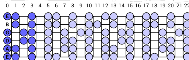
E Locrian
