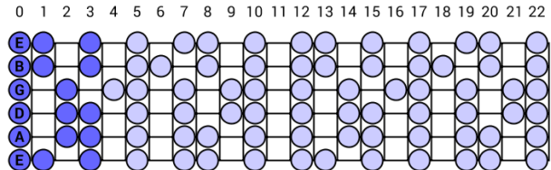
E Phrygian
