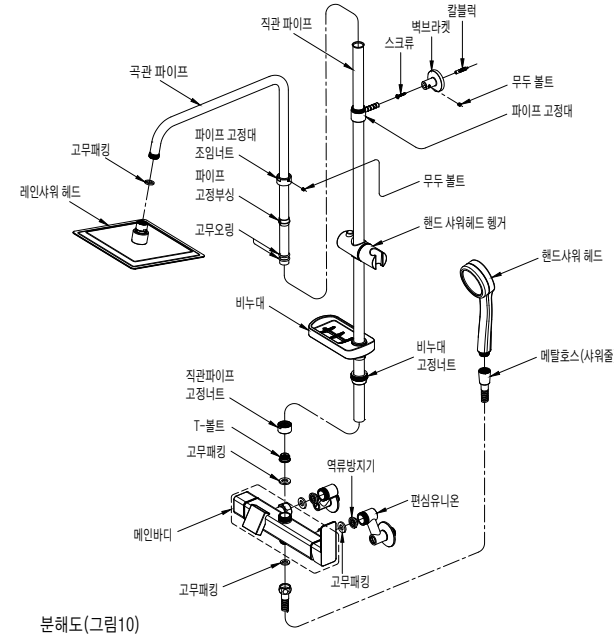
분해도(그림10)
