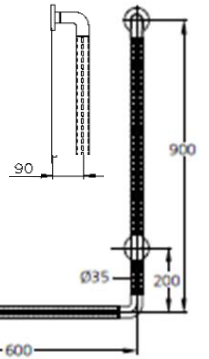
다용도 손잡이 (KPC4500W) - 우측용
