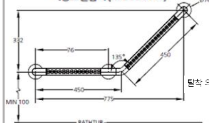
다용도 손잡이 (KPB6500W)
