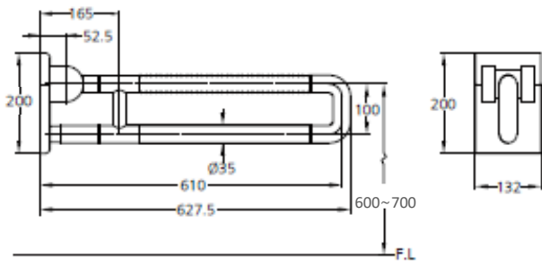
가동식 손잡이 (KPC2200W) - 상, 하
