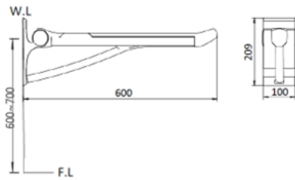
가동식 손잡이 (KPC2500W) - 상, 하
