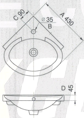
구석 붙임 세면기 L-1802(L910)
