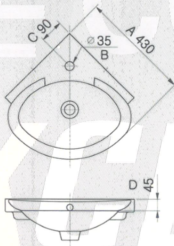
구석 붙임 세면기 L-1803F(L910)
