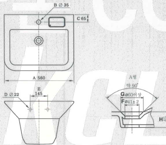
평면 붙임 세면기 L-307UD(L610)
