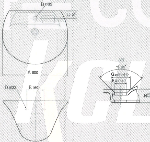
평면 불임 세면기 L-354UD(L610)
