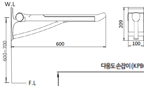
가동식 손잡이 (KPC2500W) - 상, 하
