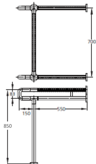
세면기용 손잡이 (KPL1000W)
