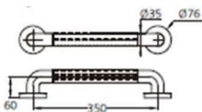
다용도 손잡이 (KPB6000W) - L=350mm
