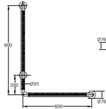
다용도 손잡이 (KPC4000W) - 좌측용
