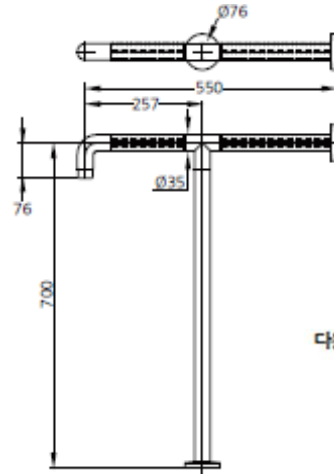
다용도 손잡이 (KPC4000W) - 좌측용
