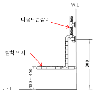
탈착 의자 (KPB4700W)
