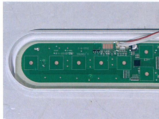
시험 후 제품 내부 사진 (6)
